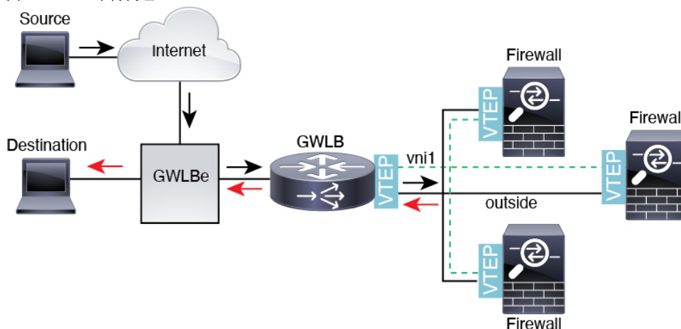
图 15: Geneve 单臂代理
