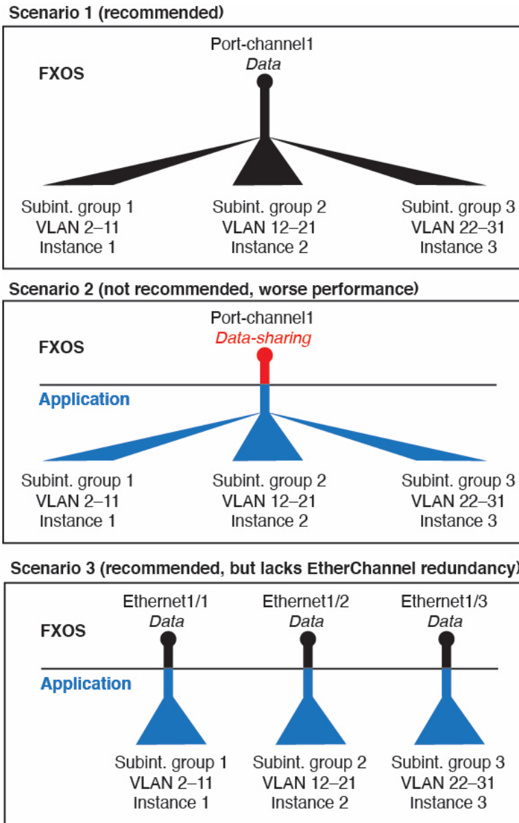
图 1: 机箱中的 VLAN 与实例
