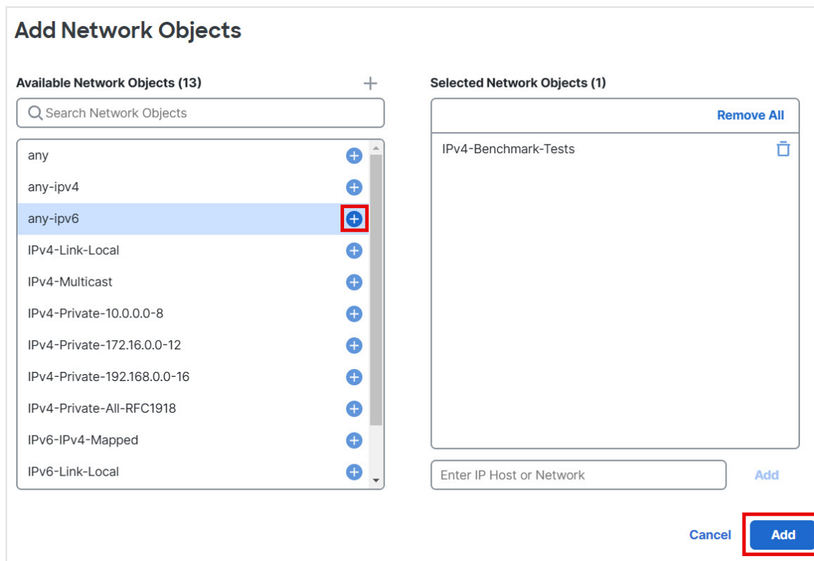
图 52: 网络对象
