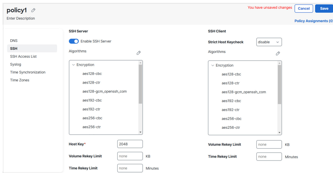
图 50: SSH
