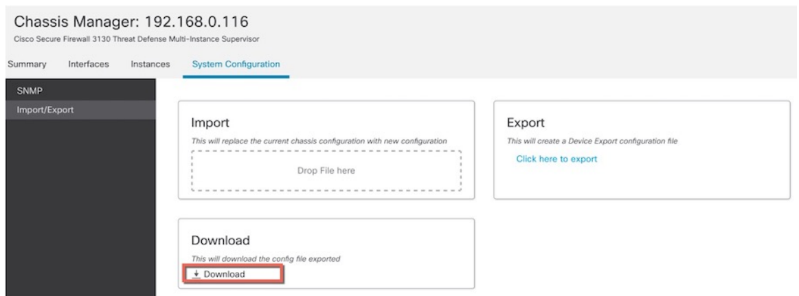
图 43: 下载
