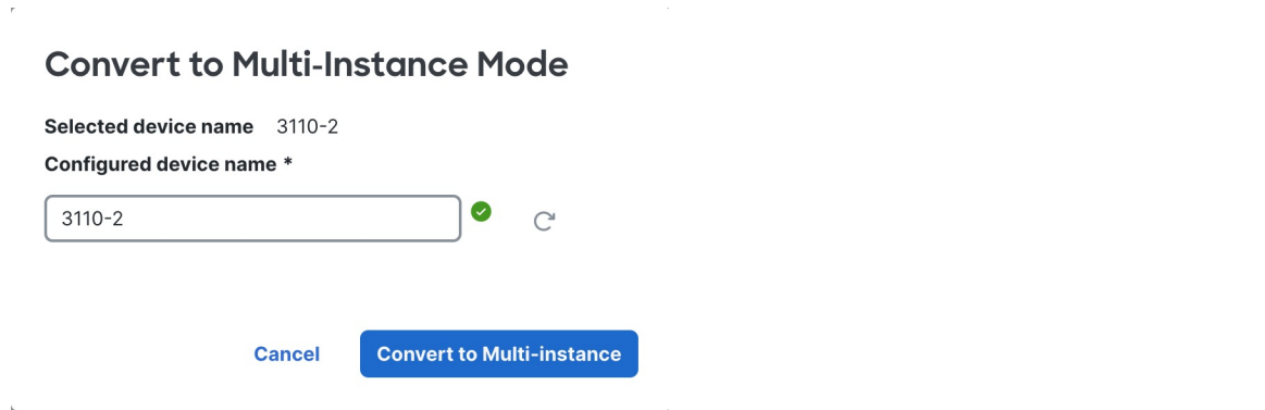
图 15: 重命名机箱
