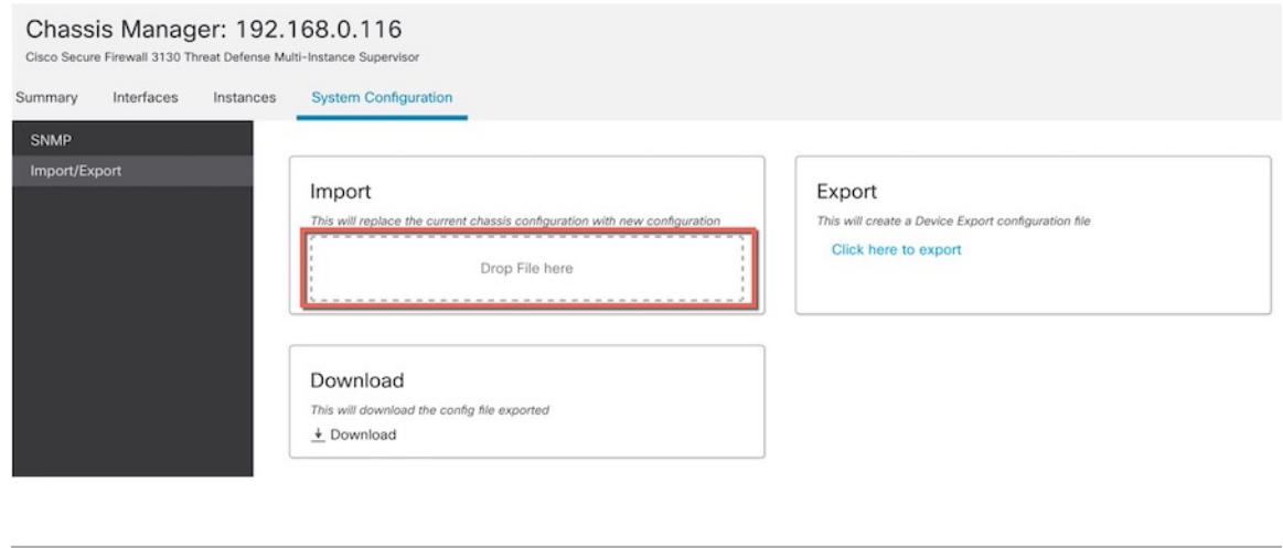
图 44: 导入
