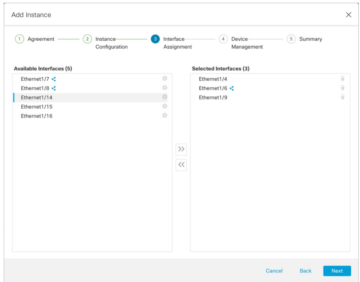
图 35: 接口分配
