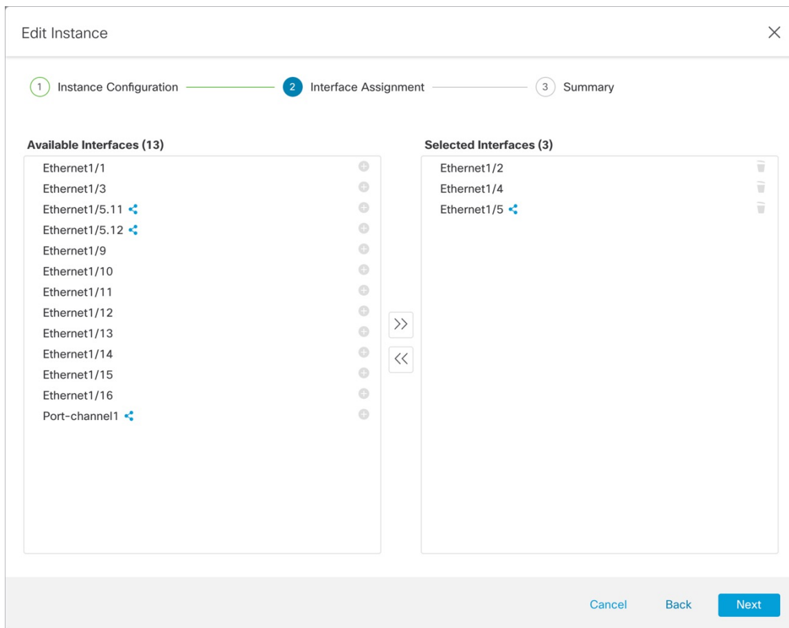
图 62: 接口分配
