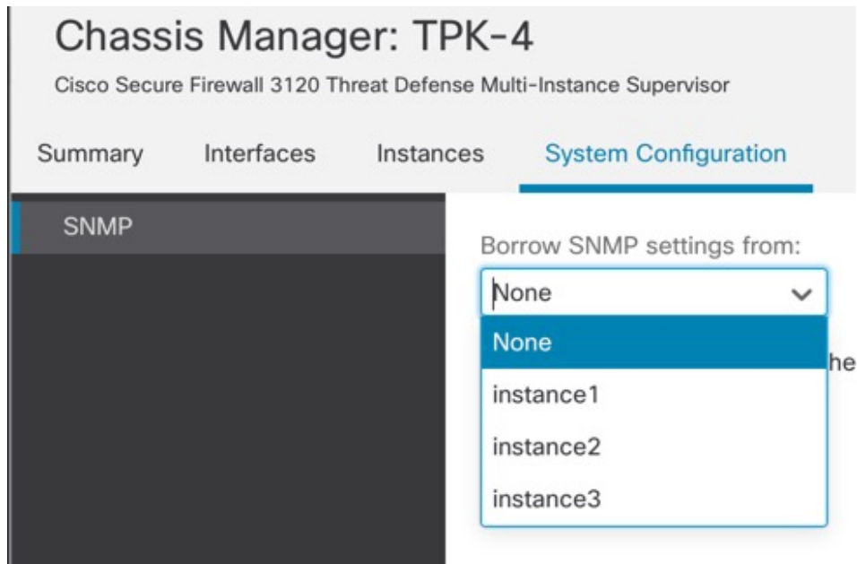
图 39: SNMP
