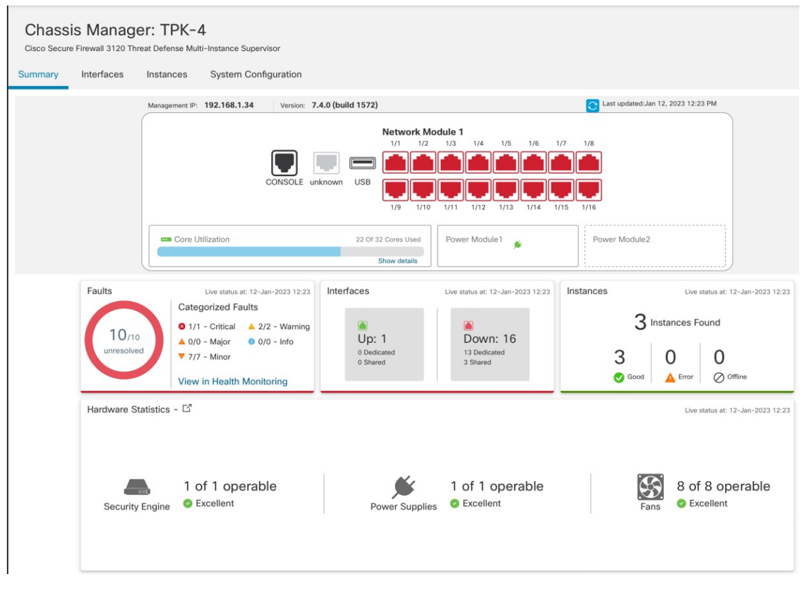
图 16: 机箱摘要
