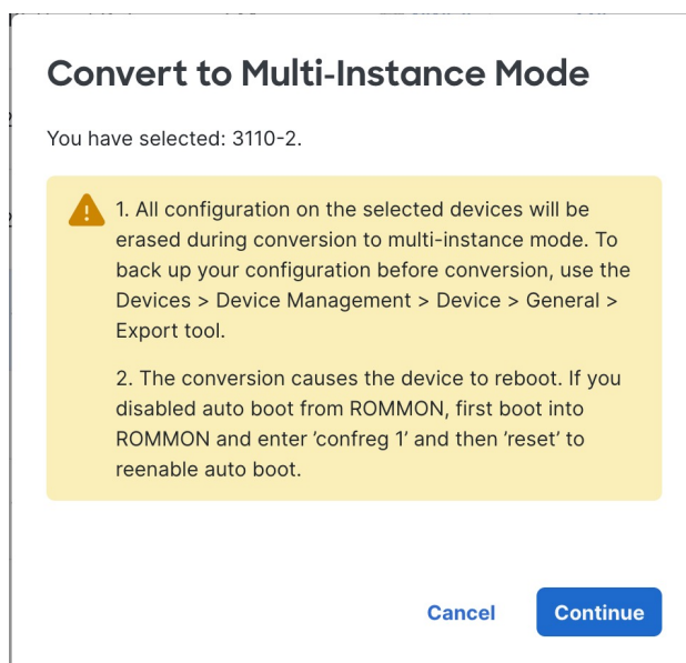
图 14: 转换确认
