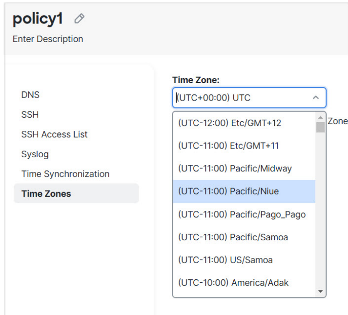
图 59: 时区
