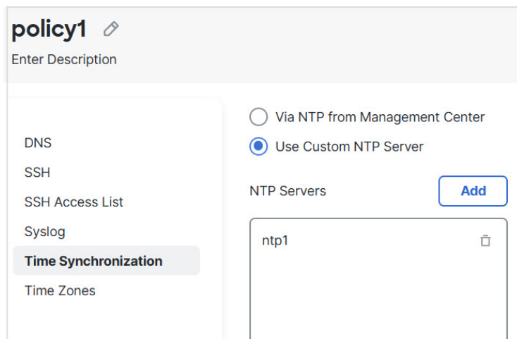
图 56: 时间同步
