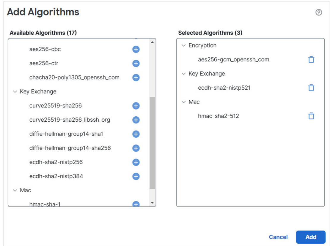
图 49: 添加算法
