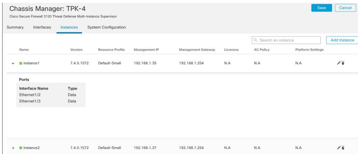
图 61: 实例
