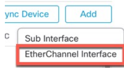
图 23: 添加 EtherChannel
