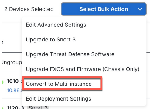
图 13: 批量转换
