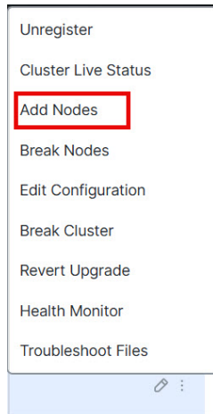
图 16: 添加节点
