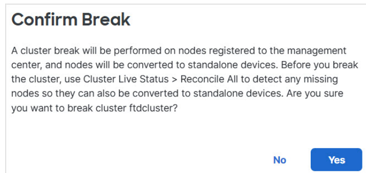
图 22: 确认中断
