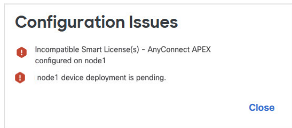
图 3: 配置问题
