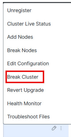
图 21: 中断集群
