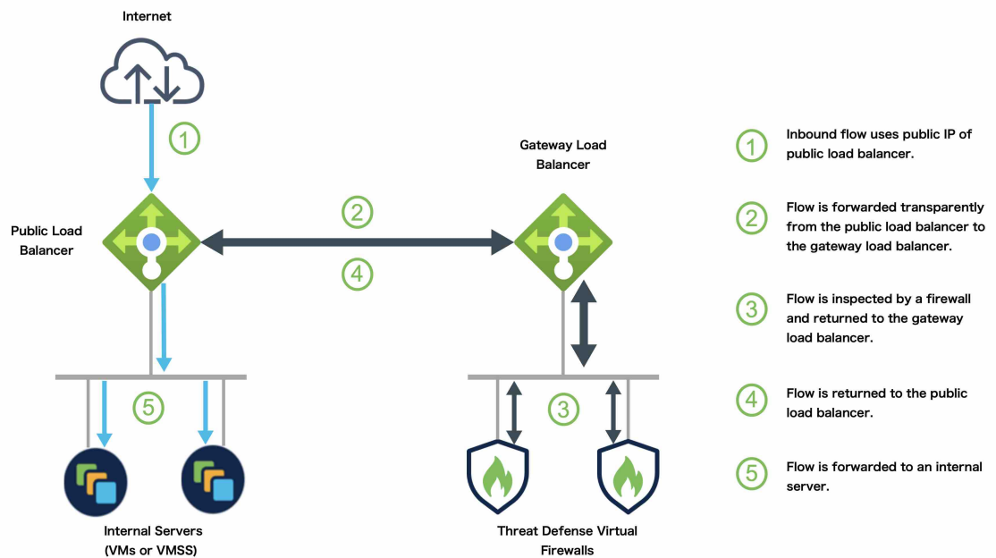
图 7: GWLB 的入站流量使用案例和拓扑
