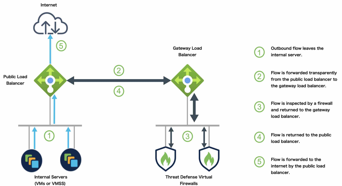
图 8: GWLB 的出站流量使用案例和拓扑
