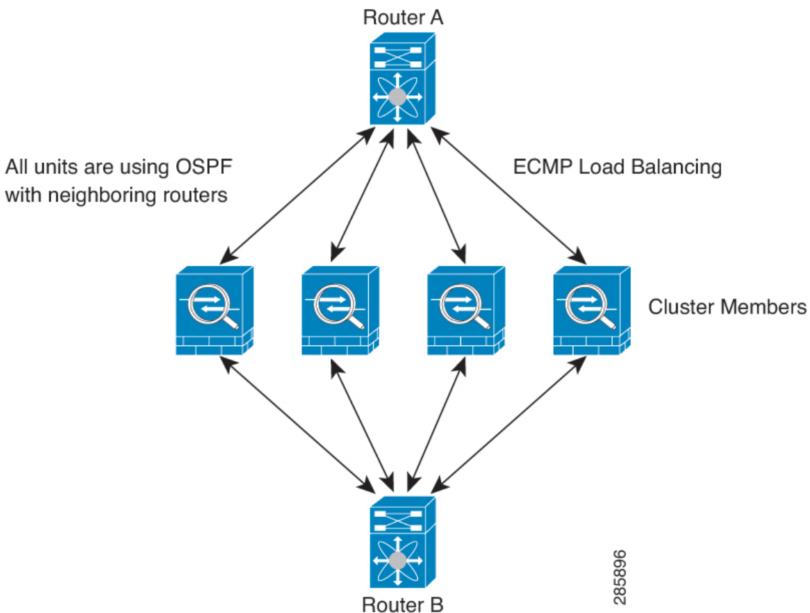
图 20: 独立接口模式下的动态路由
