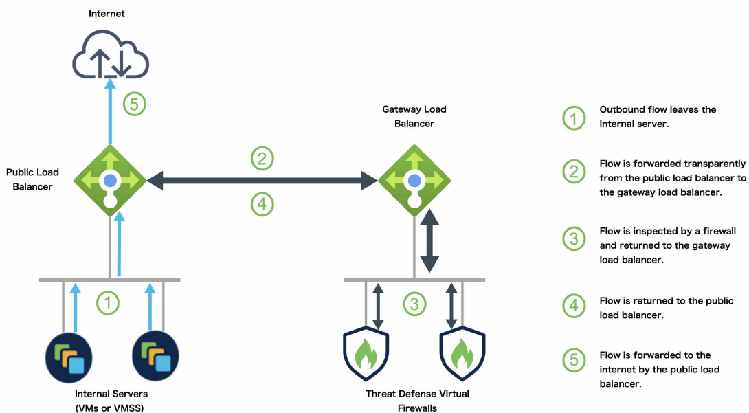
图 2: GWLB 的出站流量使用案例和拓扑
