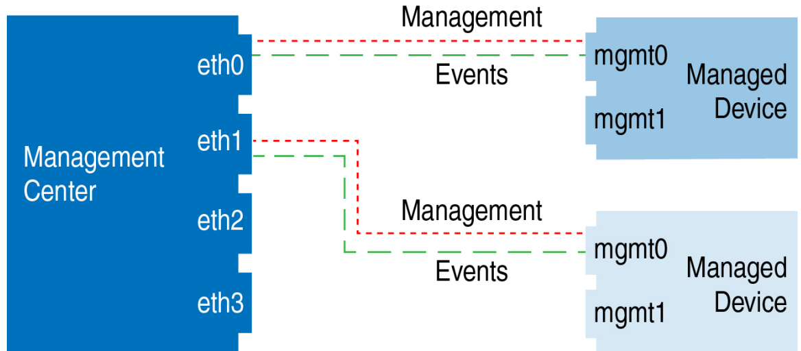
图 8: Cisco Secure Firewall Management Center 上的多个管理接口
