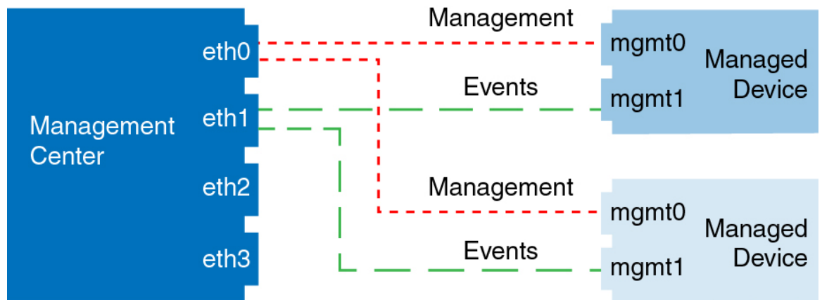
图 9: Cisco Secure Firewall Management Center 和托管设备上的单独事件接口
