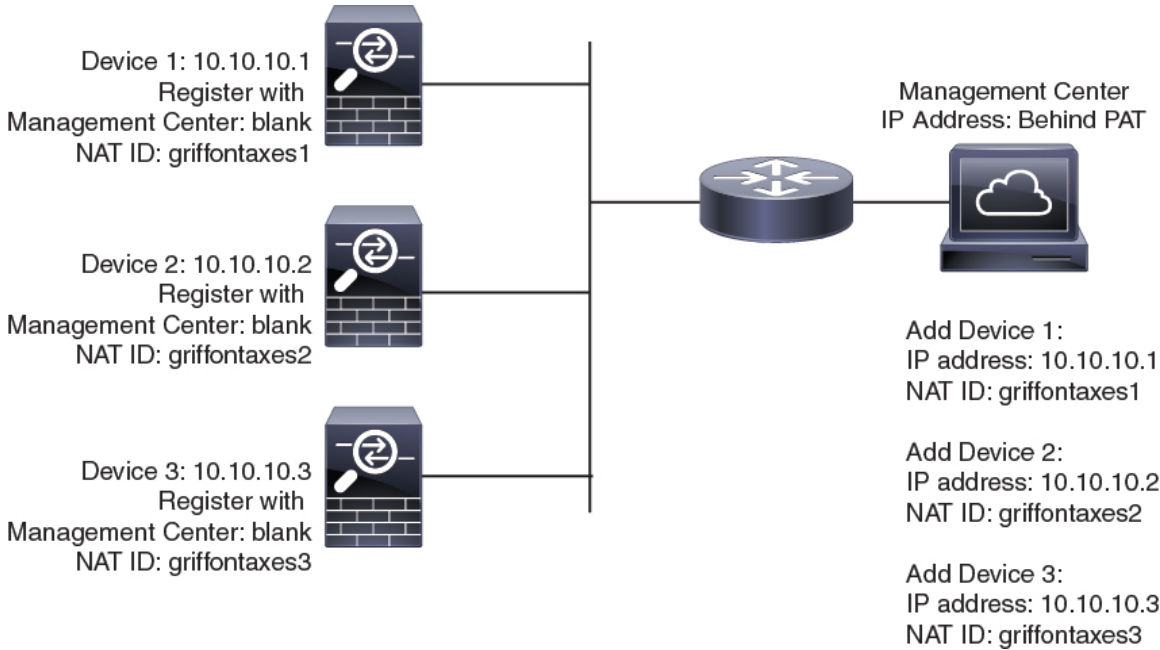
图 6: PAT 后的 FMC NAT ID
