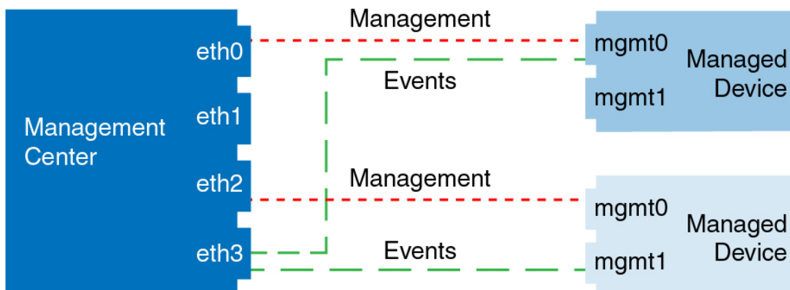
图 10: 混合管理和事件接口用法
