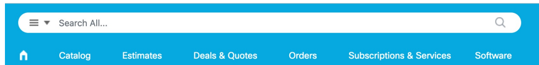
图 26: 许可证搜索
