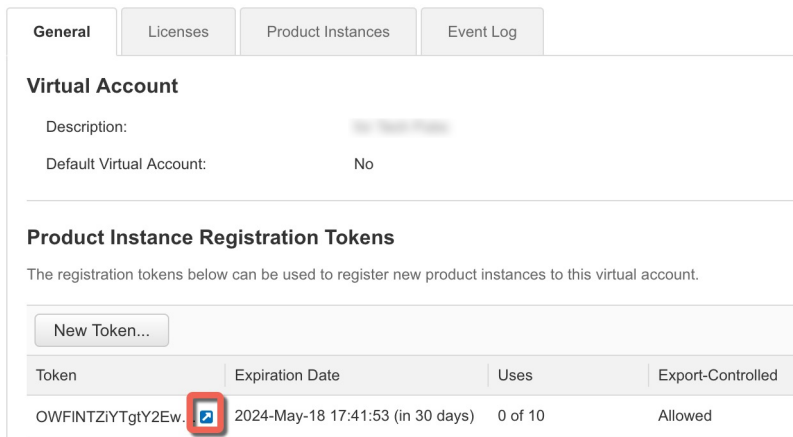
图 29: 复制令牌
