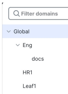
图 25: 更改为子域
