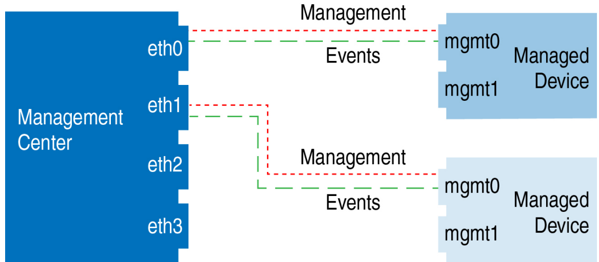
图 9: Cisco Secure Firewall Management Center 上的多个管理接口
