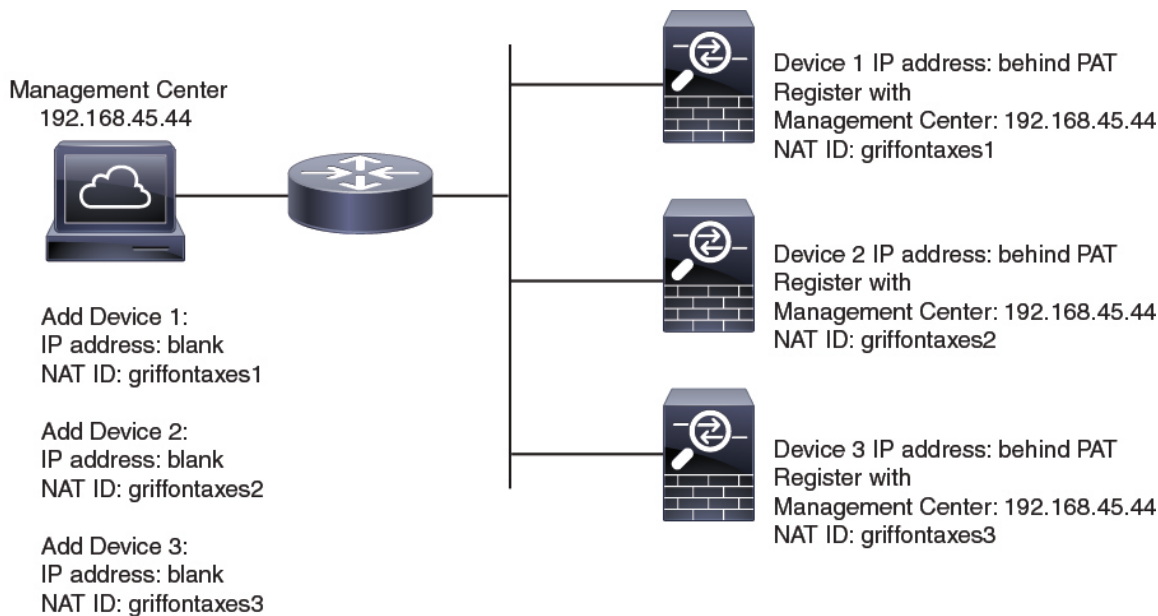
图 6: PAT 后的托管设备 NAT ID
