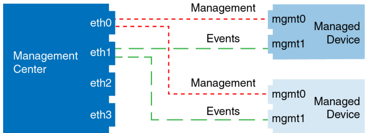
图 10: Cisco Secure Firewall Management Center 和托管设备上的单独事件接口
