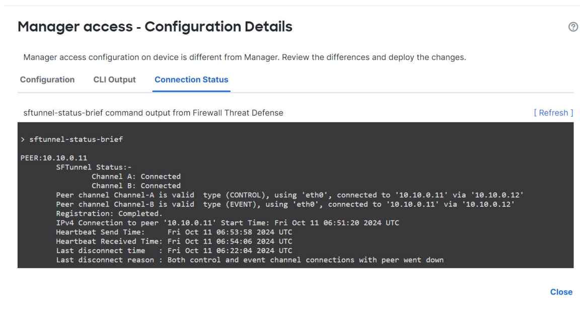
图 16: 连接状态
