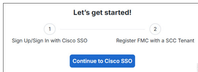
图 2: 欢迎页面
