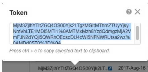
图 29: 复制令牌
