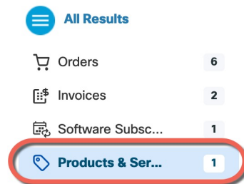
图 27: 结果
