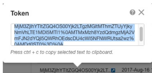
图 4: 复制令牌
