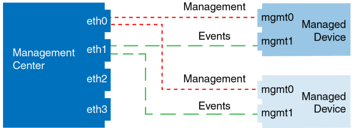
图 9: Secure Firewall Management Center 和托管设备上的单独事件接口
