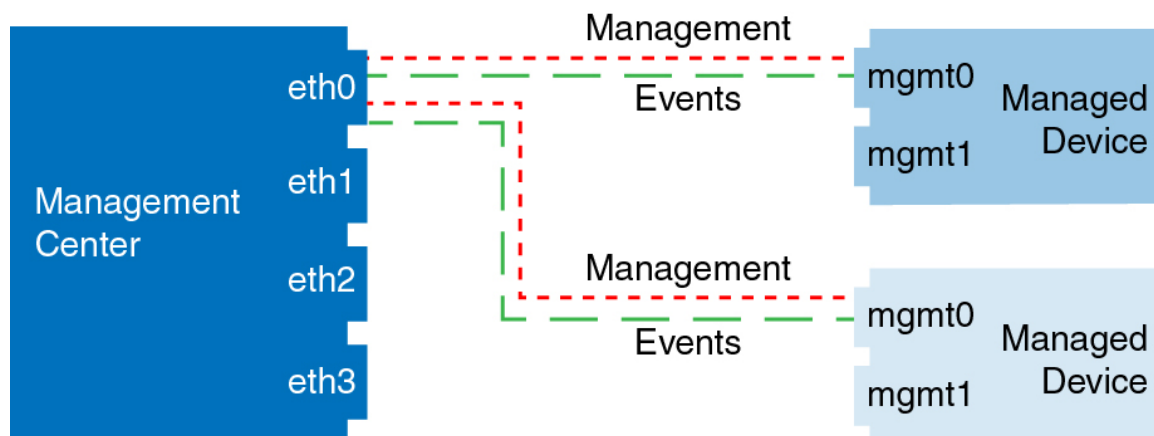
图 7: Secure Firewall Management Center 上的单个管理接口
