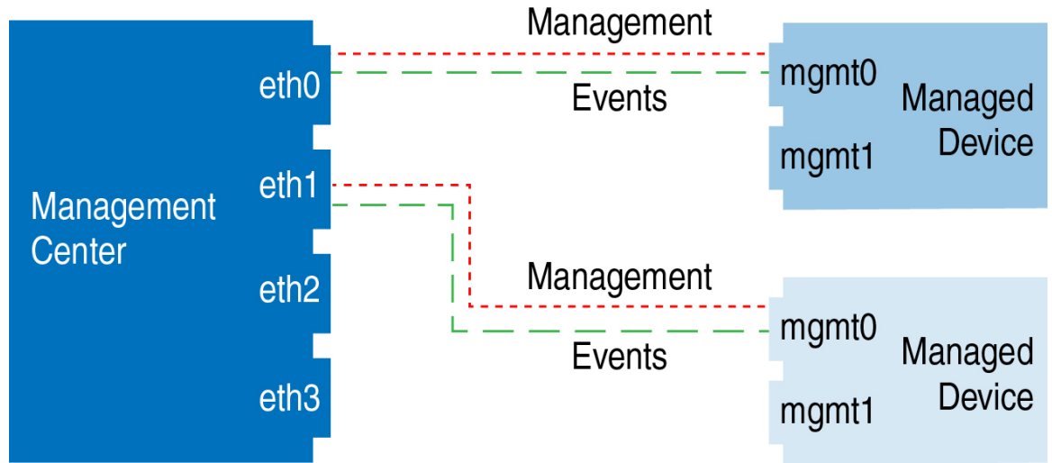
图 8: Secure Firewall Management Center 上的多个管理接口
