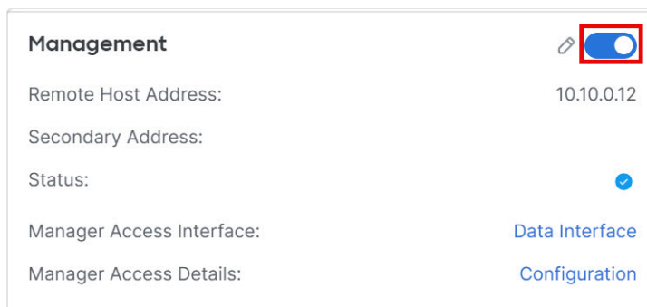
图 11: 禁用管理
