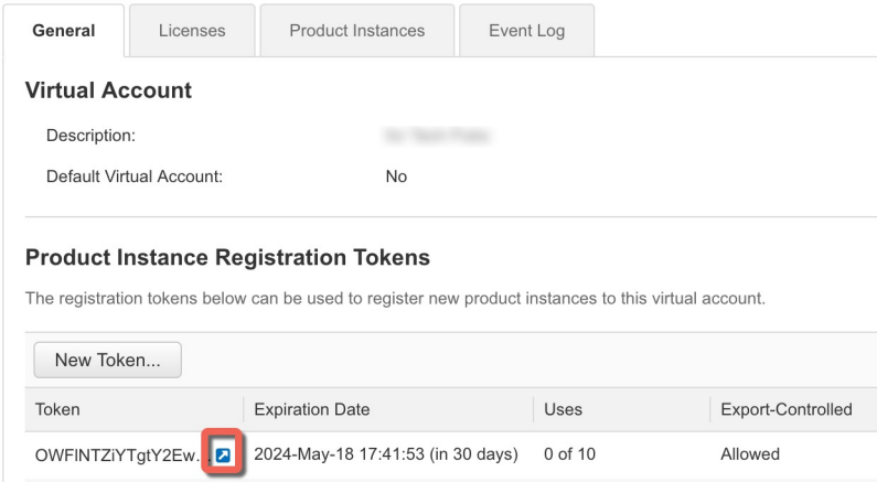
图 4: 复制令牌
