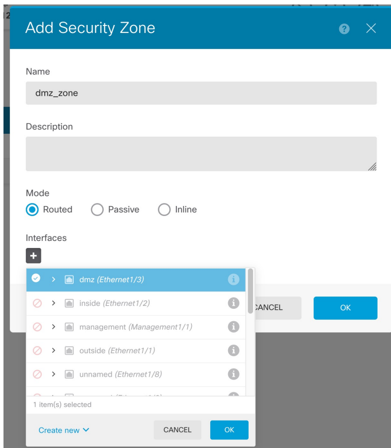
图 6: 安全区域对象
