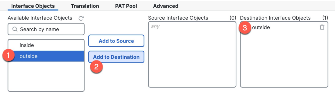
图 15: 接口对象
