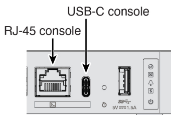
图 5: 控制台端口
