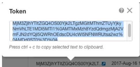
图 5: 复制令牌
