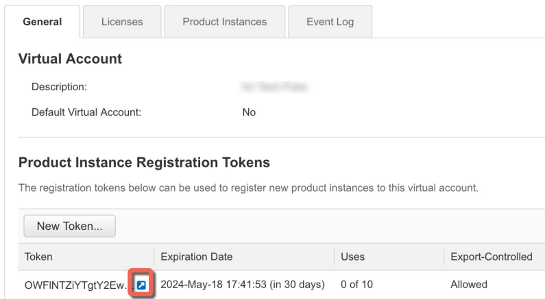
图 5: 复制令牌
