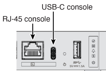
图 3: 控制台端口
