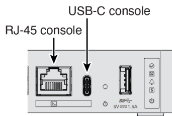
图 4: 控制台端口
