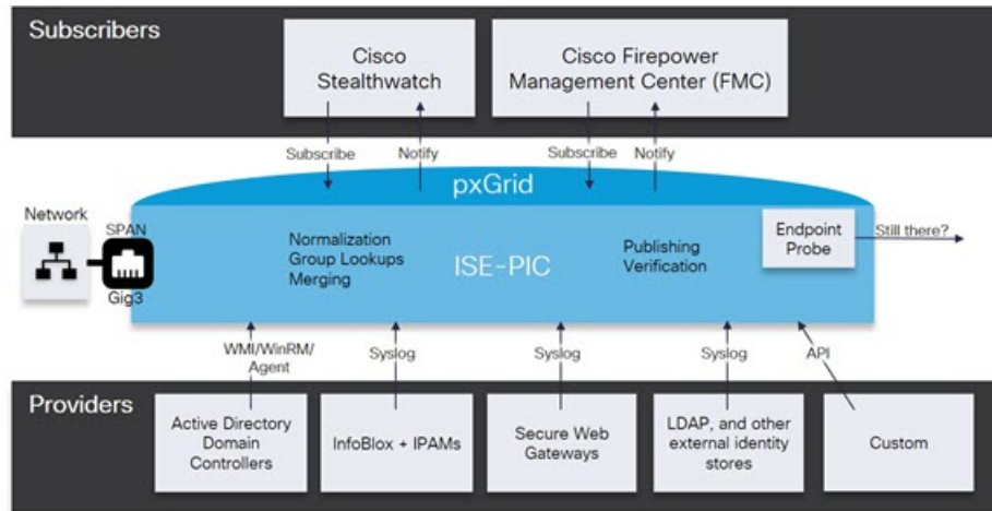
图 9: 概要流程
