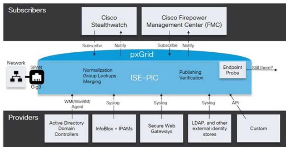
图 13: 被动身份服务流
