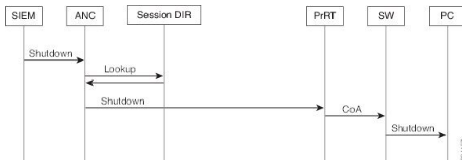
图 11: ANC 关闭流程
