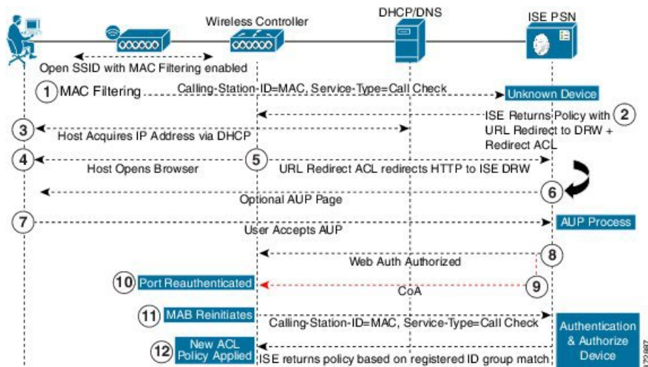
图 13: 无线设备注册 Web 身份验证流程
