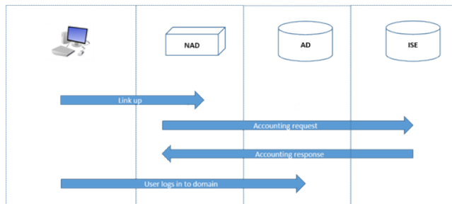
图 21: Easy Connect 可见性模式流程
