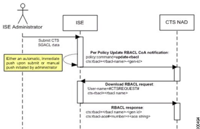
图 50: 更新 SGACL 内容流程
