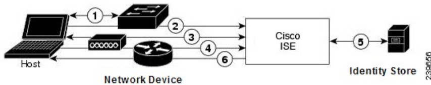
图 46: 使用 EAP 的基于 RADIUS 的身份验证
