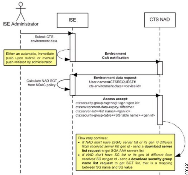
图 49: 环境 CoA 通知流程
