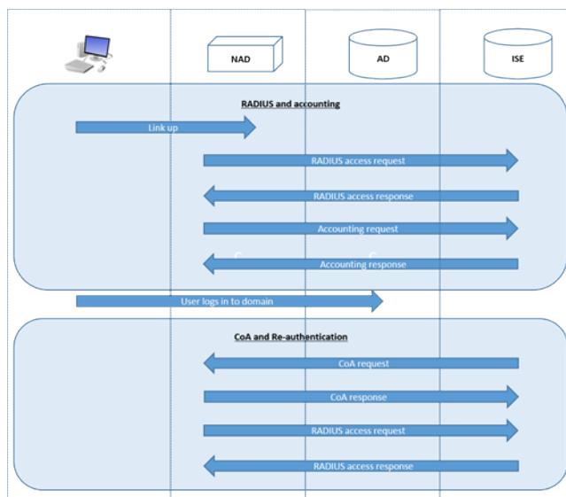
图 20: Easy Connect 实施模式详细流程
