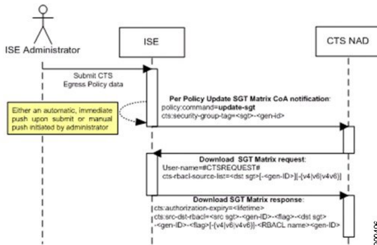
图 52: 更新 SGT 矩阵 CoA 流程
