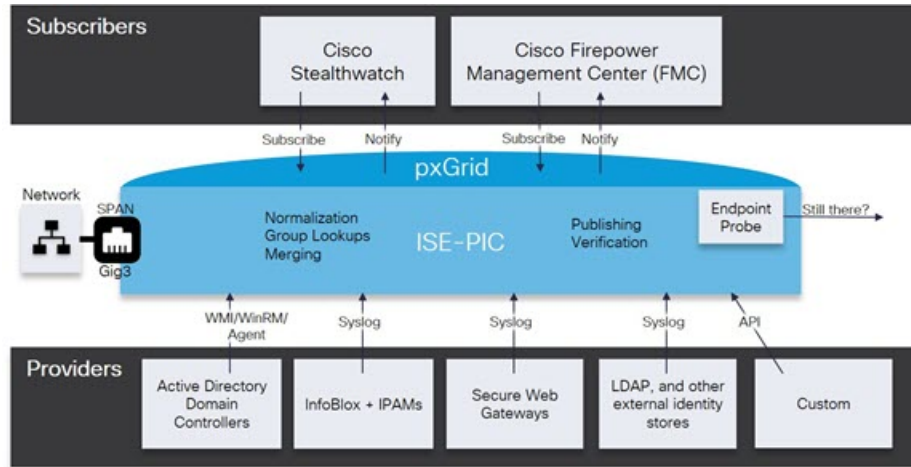
图 26: 被动身份服务流
