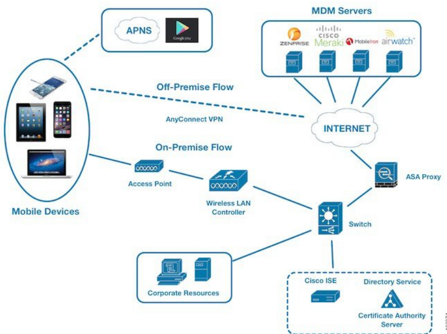
图 32: MDM 与思科 ISE 的互通性
