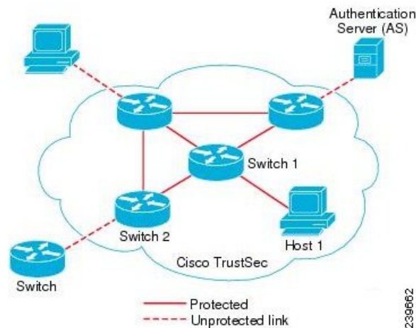
图 47: TrustSec 架构
