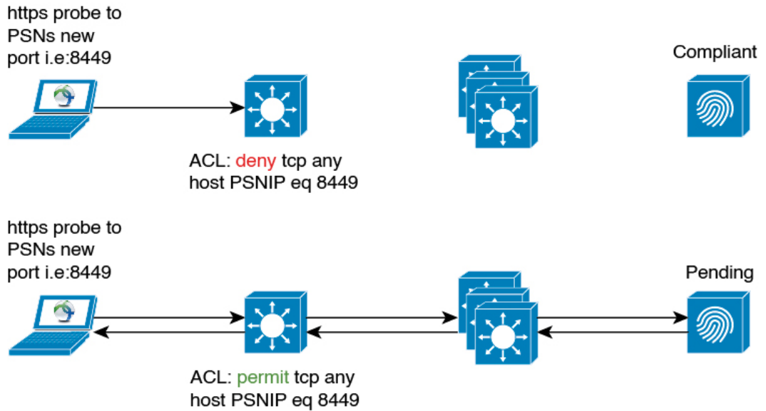
图 64: 双向安全评估流程
