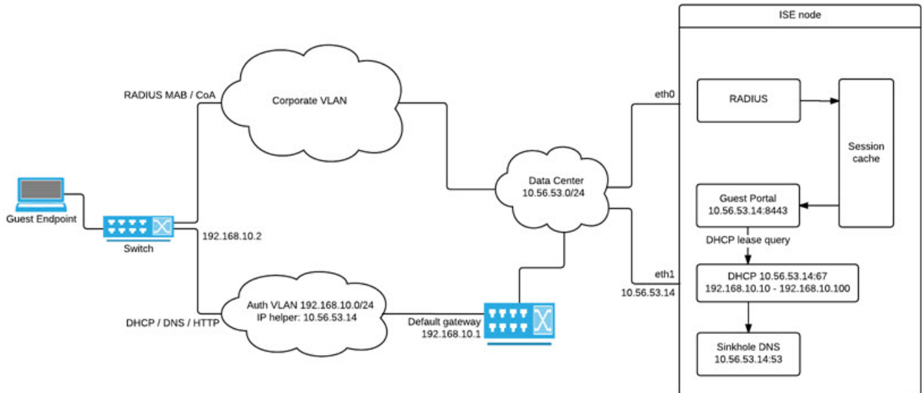
图 31: 配置有 IP 助手的身份验证 VLAN
