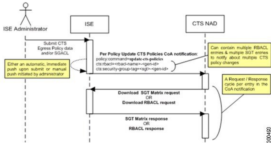
图 51: 策略 CoA 通知流程
