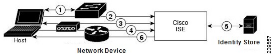
图 45: 不使用 EAP 的基于 RADIUS 的身份验证
