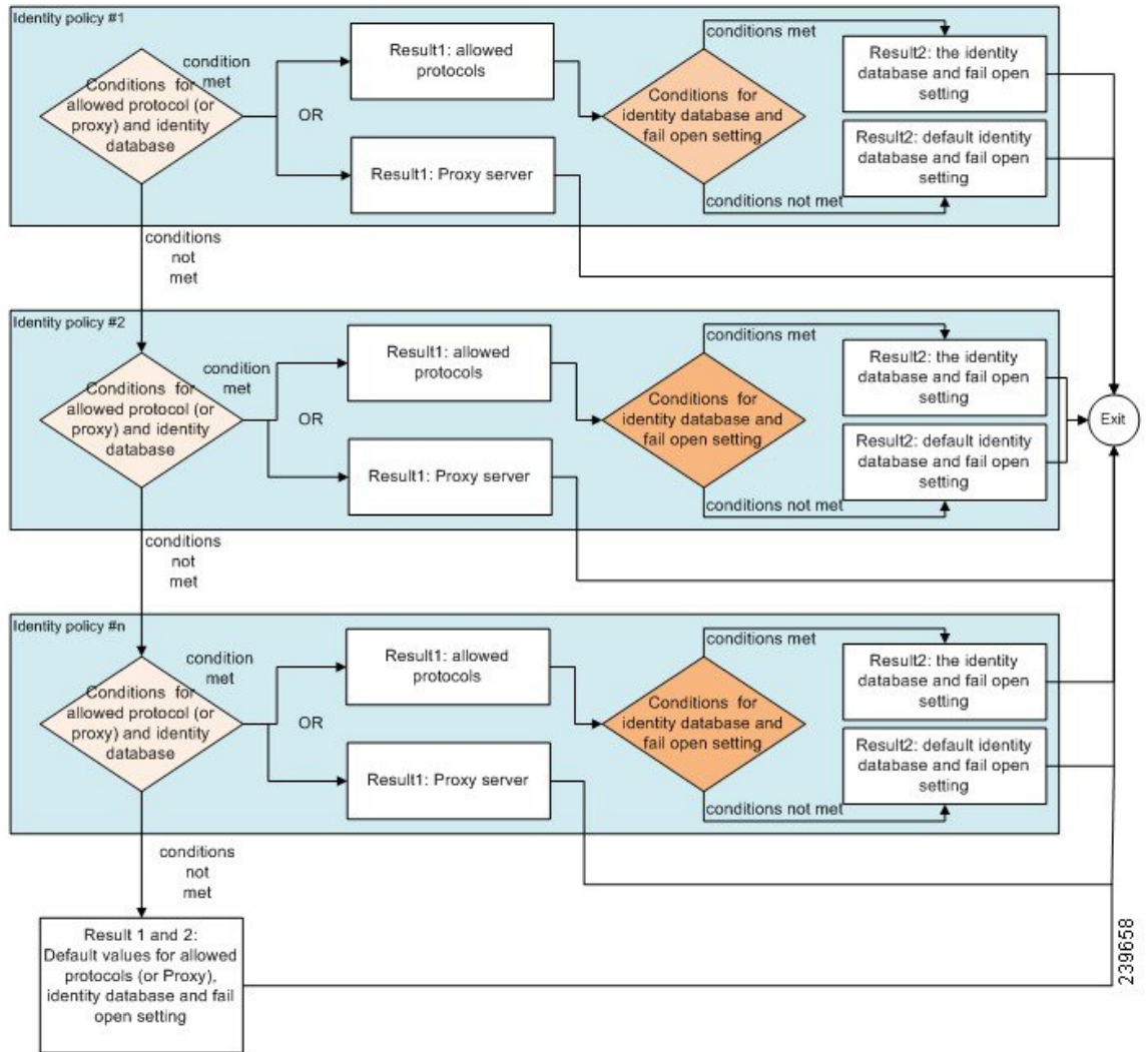
图 39: 身份验证策略流
