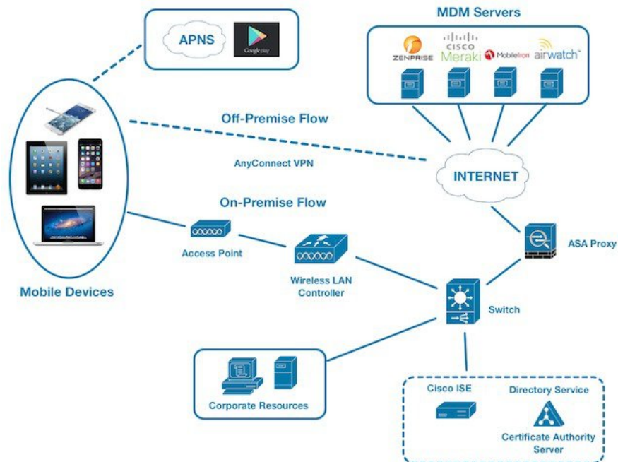
图 3: MDM 与思科 ISE 的互通性
