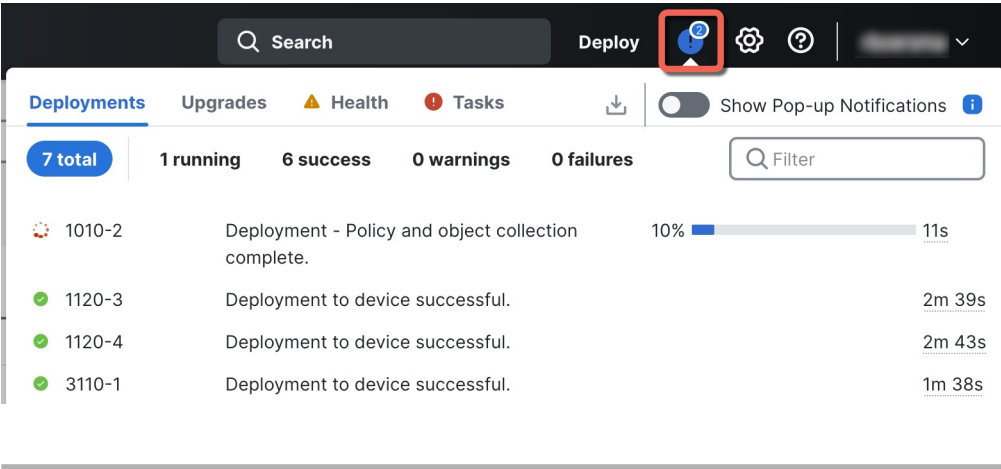
图 43: 部署状态
