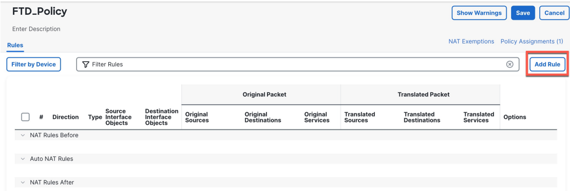
图 29: NAT 策略
