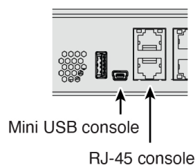
图 3: 控制台端口
