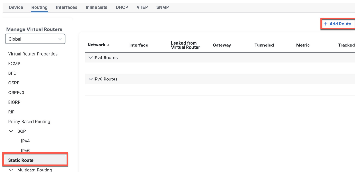
图 26: 静态路由
