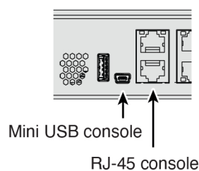
图 5: 控制台端口
