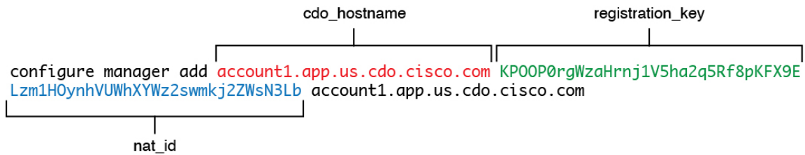
图 27: 配置管理器添加命令组件
