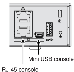
图 3: 控制台端口
