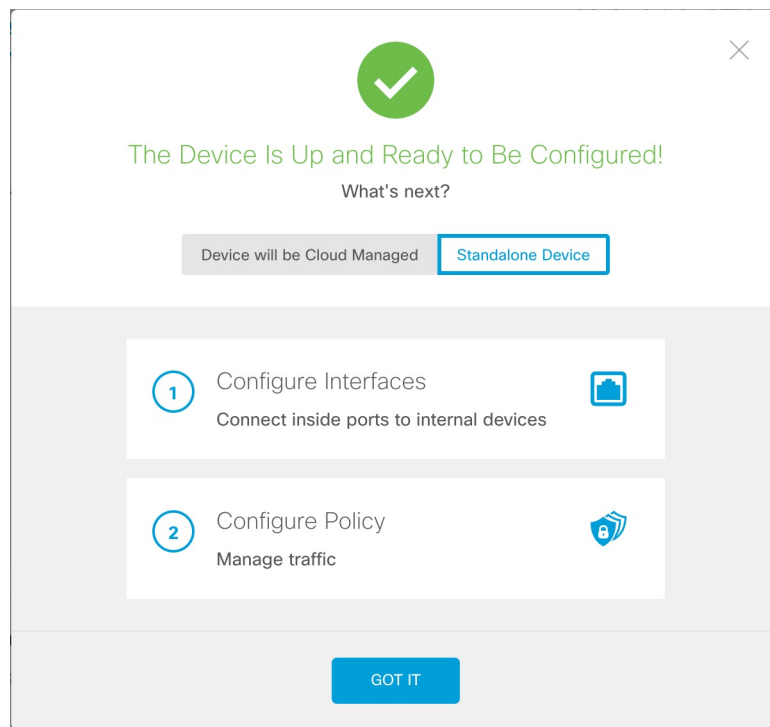
图 25: 后续操作
