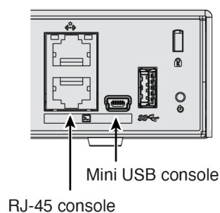
图 2: 控制台端口
