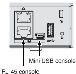
图 4: 控制台端口
