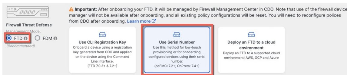
图 8: 使用序列号
