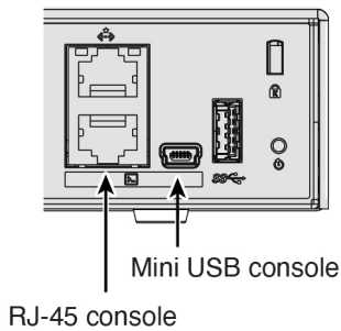
图 2: 控制台端口
