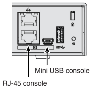
图 3: 控制台端口
