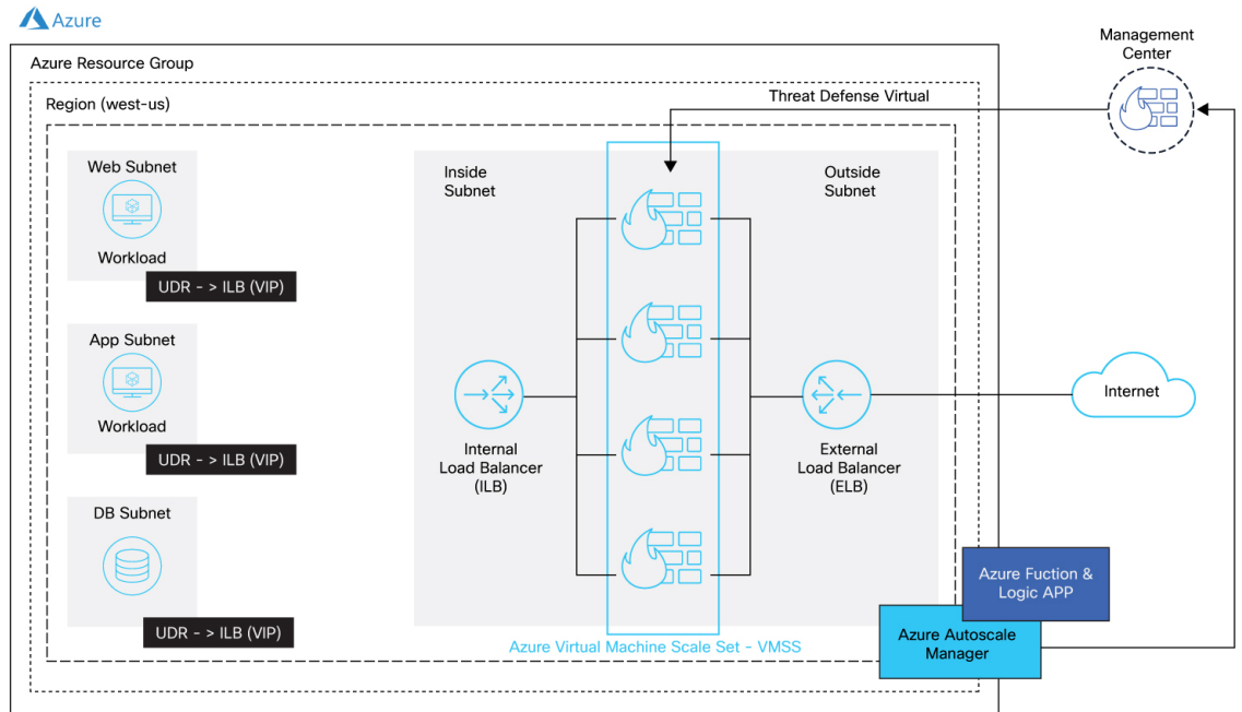
图 5: 使用三明治拓扑的 Firewall Threat Defense Virtual Auto Scale 使用案例图
