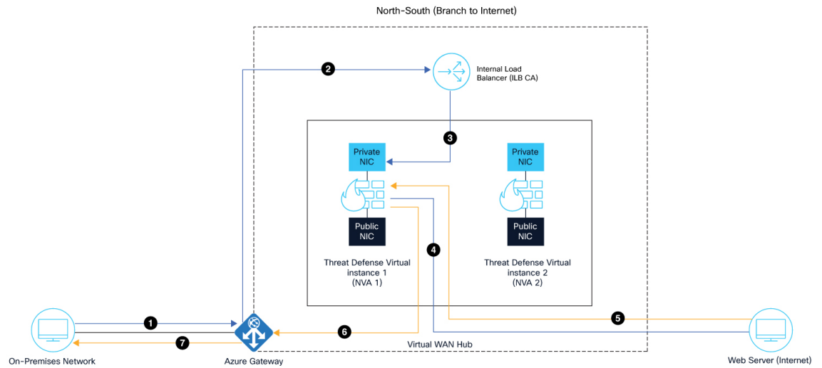
图 34: Azure 虚拟 WAN 中心中的 Firewall Threat Defense Virtual 南北流量检测拓扑
