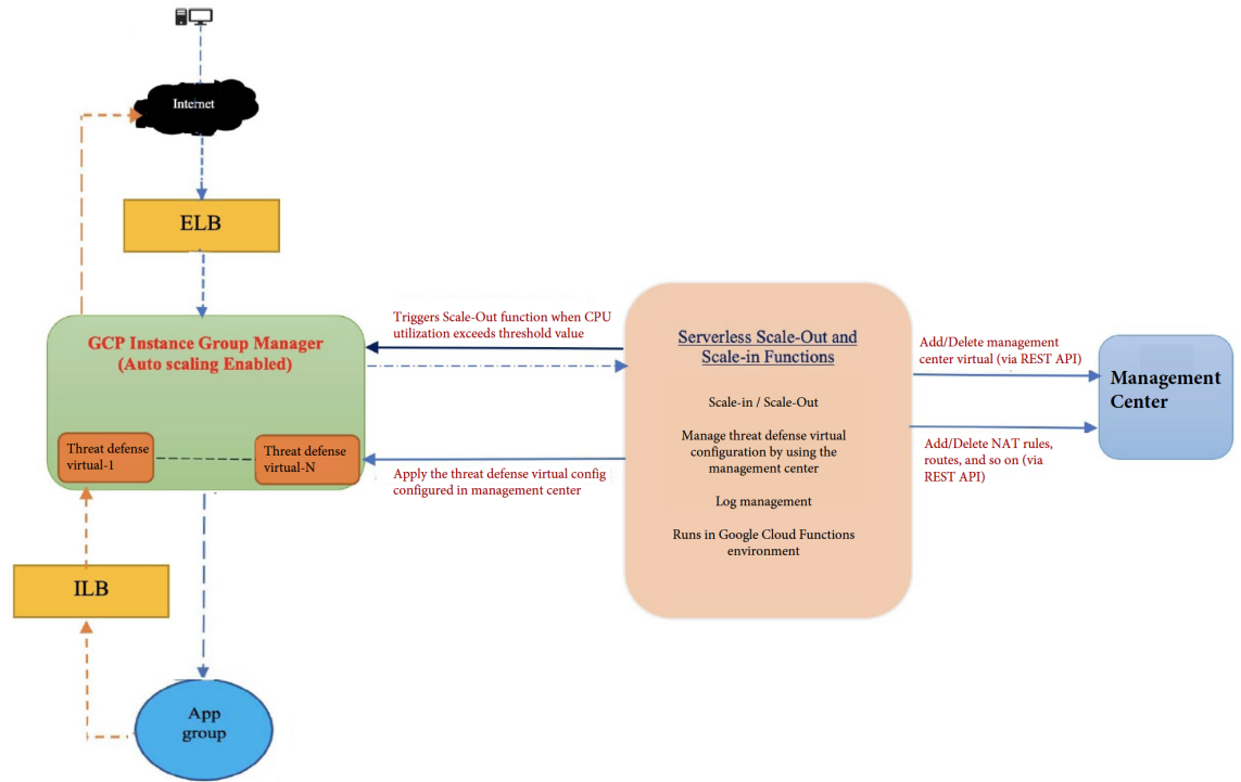
图 48: Auto Scale 解决方案概述
