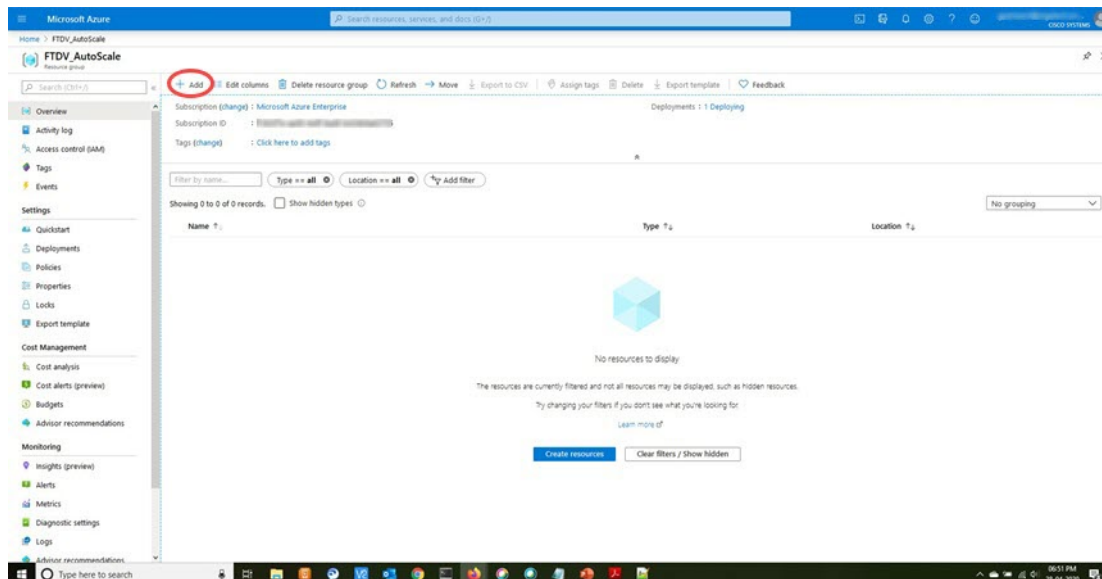
图 13: Azure 门户
