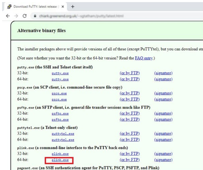
图 21: 下载 PuTTY
