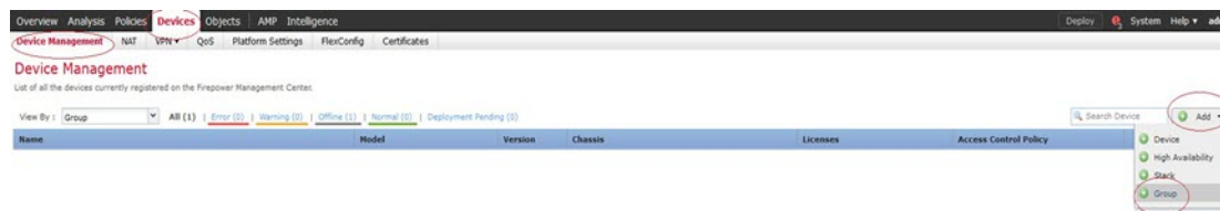
图 7: 设备管理
