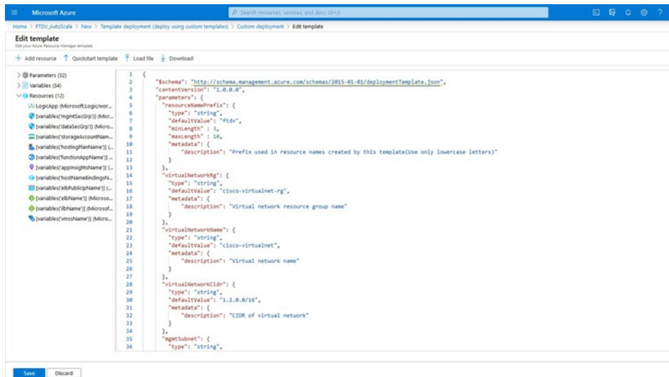
图 16: 编辑模板
