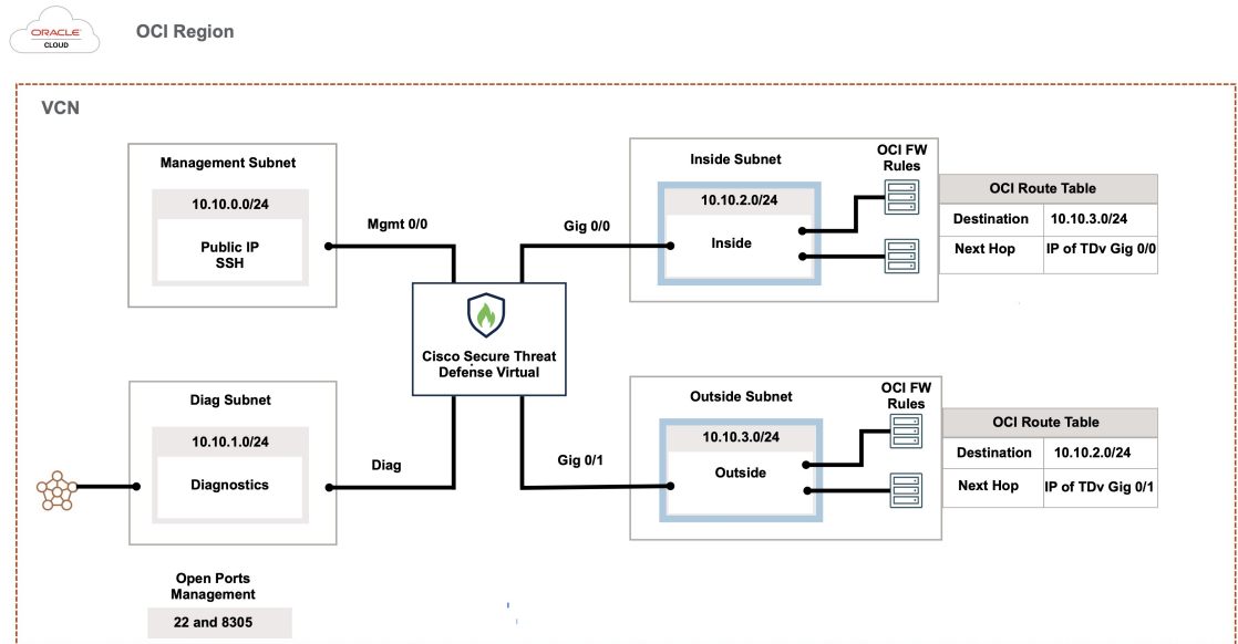
图 37: VCN 中具有四个子网的 OCI 部署示例 Firewall Threat Defense Virtual
