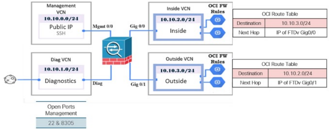
图 37: VCN 中具有四个子网的 OCI 部署示例 Firewall Threat Defense Virtual
