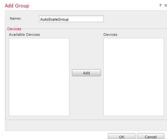
图 8: 添加设备组
