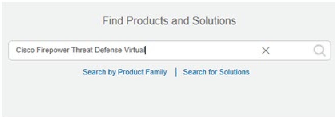
图 6: 许可证搜索
