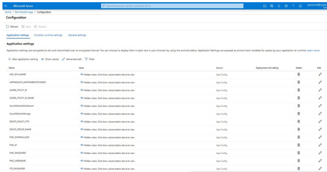
图 23: 应用设置
