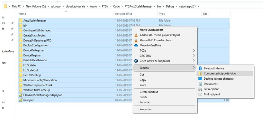
图 33: 生成 ASM_Function.zip
