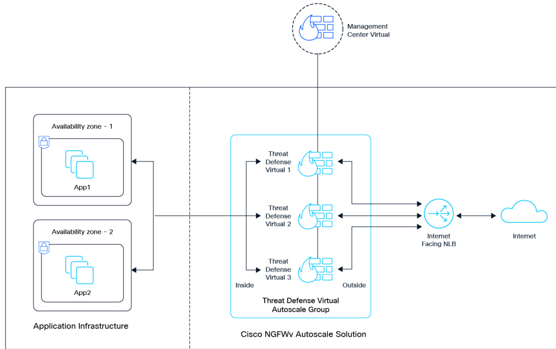
图 3: 使用 NLB 的 Firewall Threat Defense Virtual Auto Scale 解决方案
