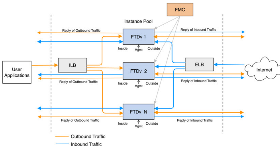
图 39: Cisco Secure Firewall Threat Defense Virtual Auto Scale 使用案例图
