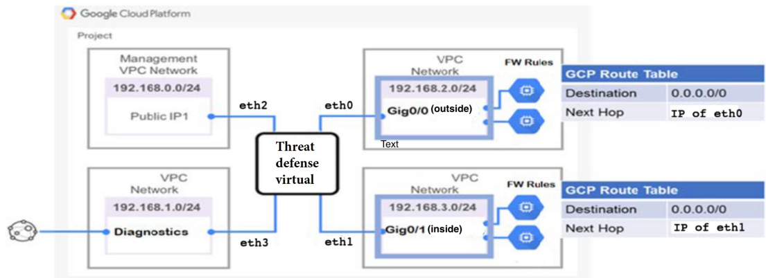
图 44: GCP 上的 Firewall Threat Defense Virtual 部署示例
