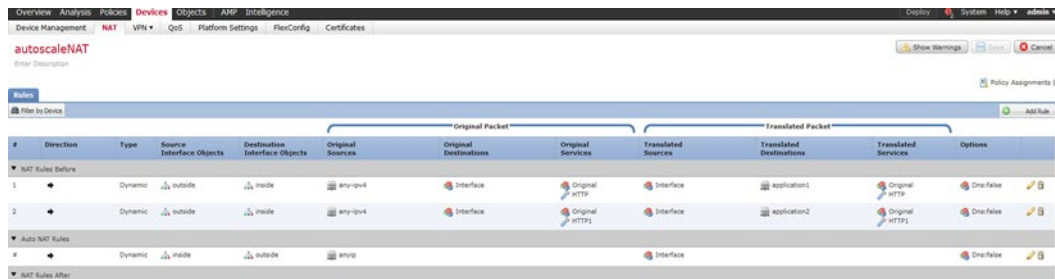
图 12: NAT 策略示例
