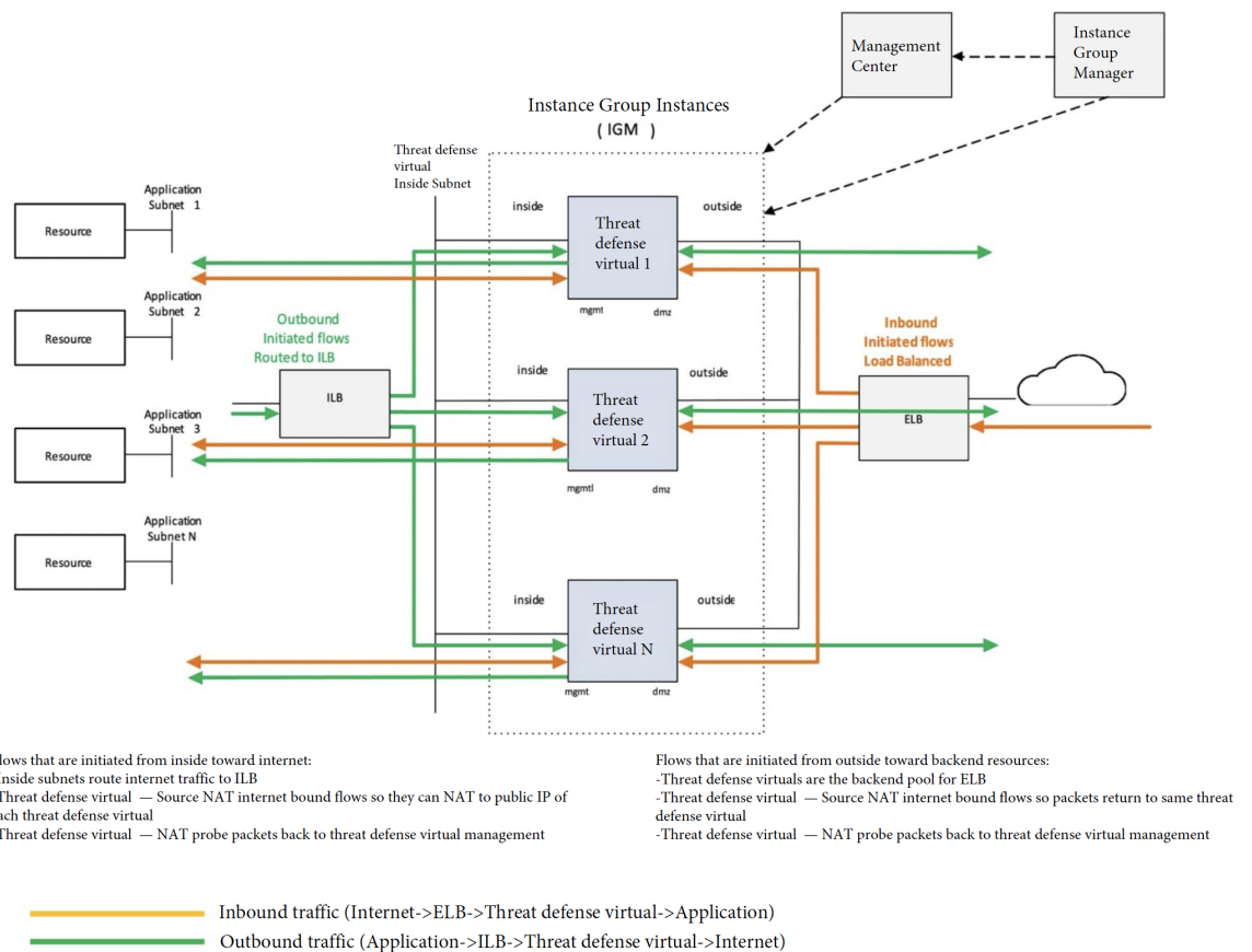
图 45: Firewall Threat Defense Virtual Auto Scale 使用案例
