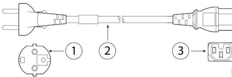
图 17: 欧洲 CAB-9K10A-EU
