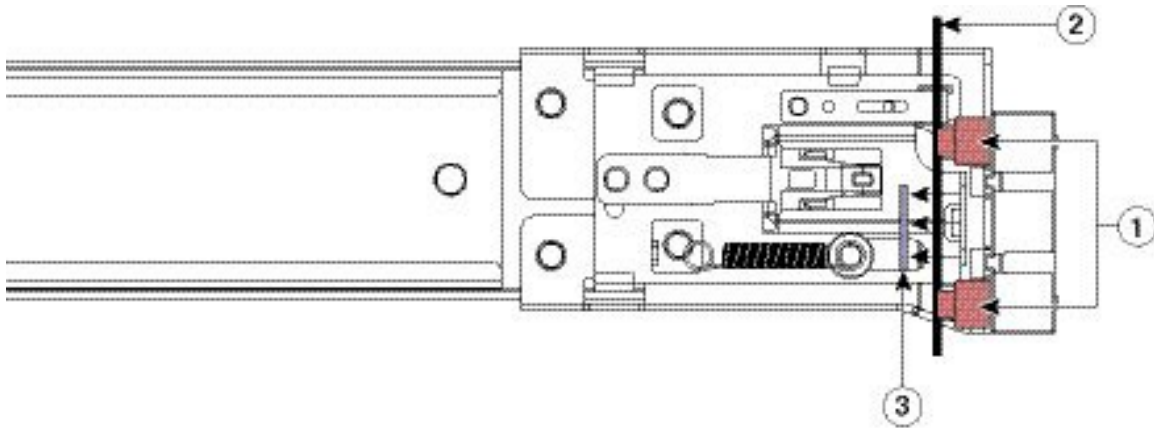
图 31: 前紧固装置，前端内侧
