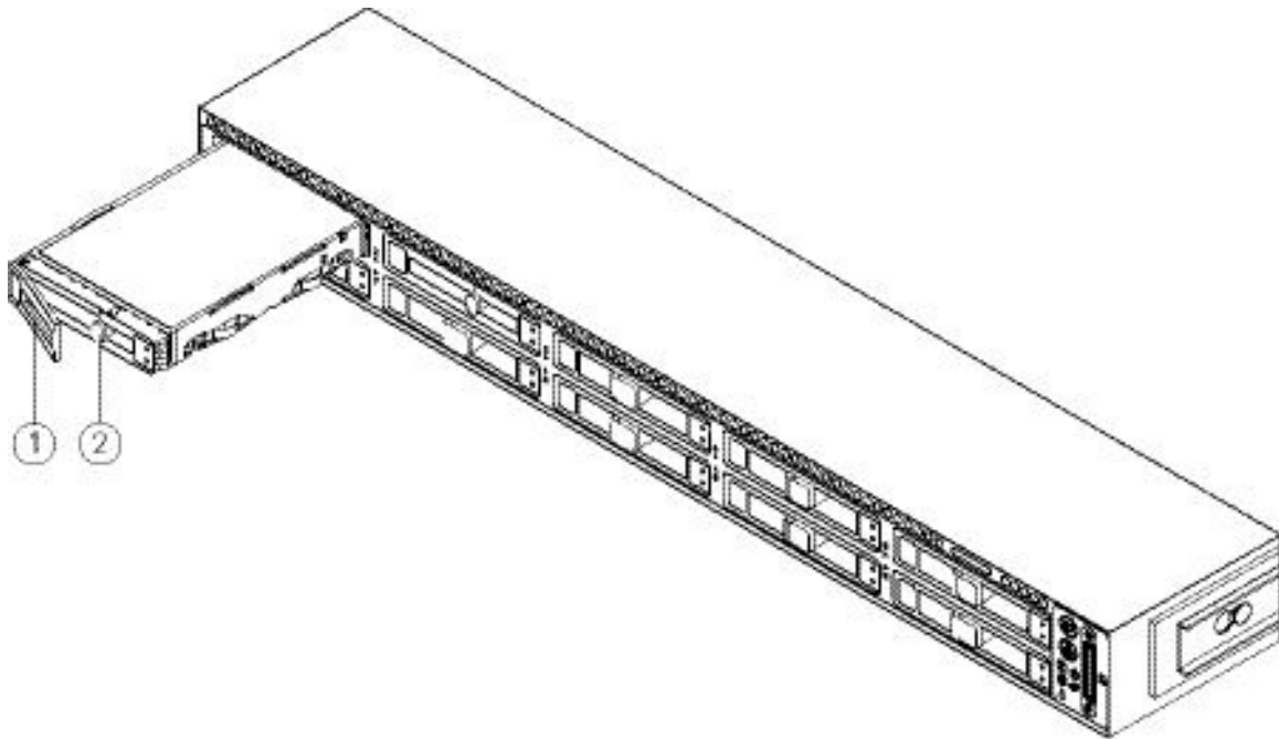
图 33: 拆卸驱动器
