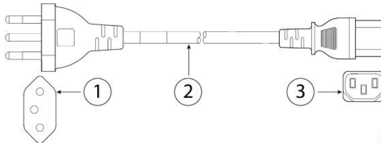
图 12: 巴西 PWR-250V-10A-BZ
