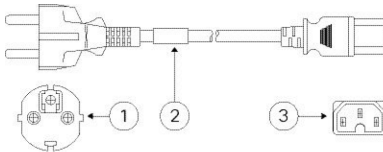
图 23: 韩国 CAB-9K10S-KOR
