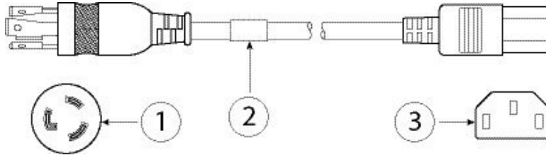
图 26: 北美 CAB-AC-L620-C13
