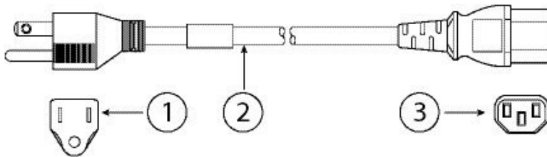
图 21: 日本 CAB-JPN-3PIN
