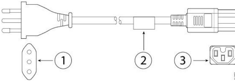
图 20: 意大利 CAB-9K10A-IT
