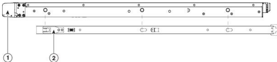
图 30: 将内滑轨固定到机箱的侧面
