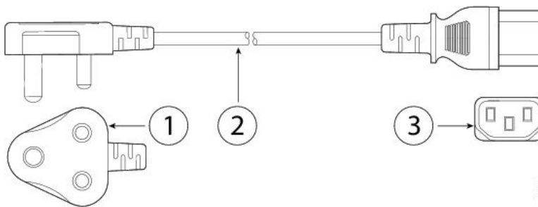
图 18: 印度 CAB-250V-10A-ID
