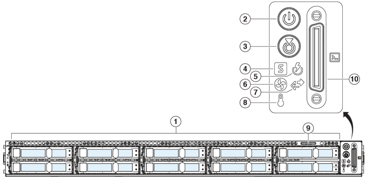
图 6: FMC 4600 前面板
