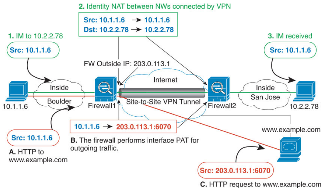
图 1: 用于站点间 VPN 的接口 PAT 和身份 NAT
