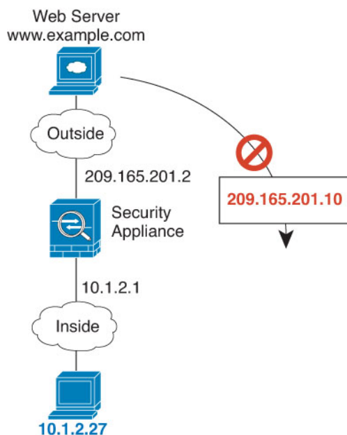
图 4: 远程主机尝试向映射地址发起连接
