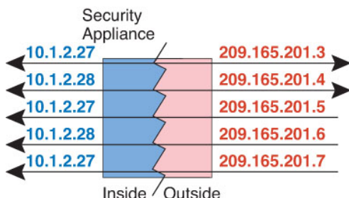
图 10: 少对多静态 NAT
