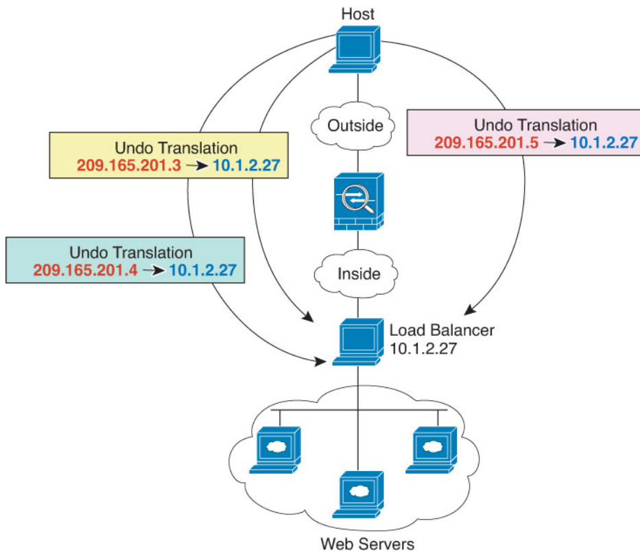
图 9: 一对多静态 NAT 示例
