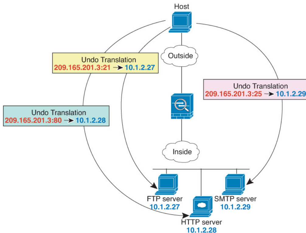
图 14: 支持端口转换的静态 NAT
