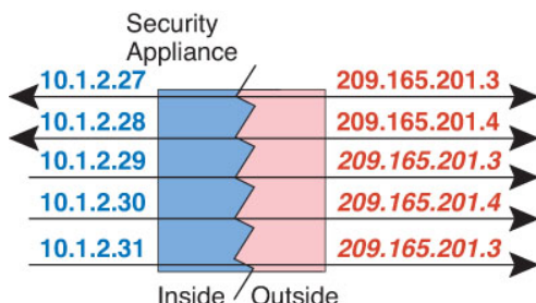
图 11: 多对少静态 NAT
