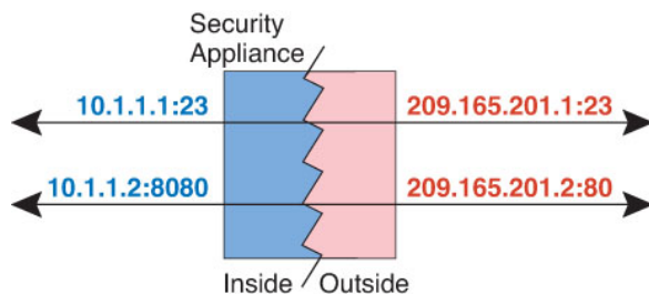
图 7: 支持端口转换的典型静态 NAT 场景
