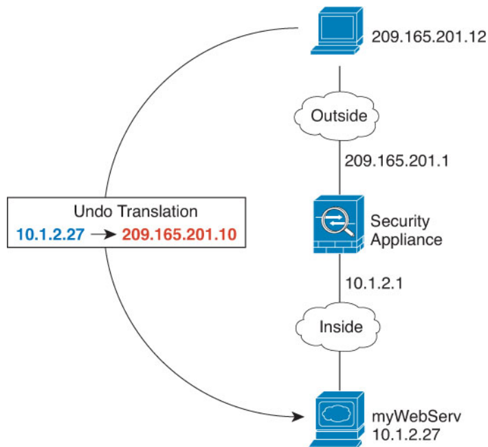
图 13: 面向内部 Web 服务器的静态 NAT
