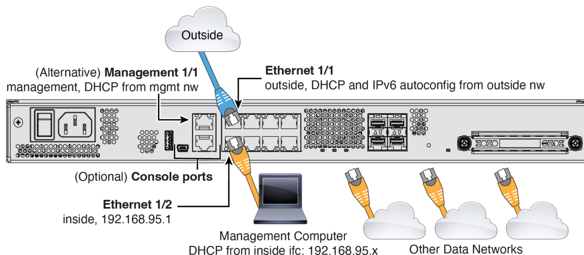
图 2: Firepower 1100 的布线
