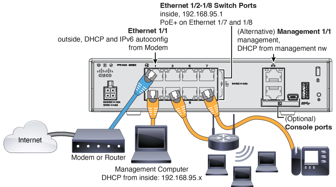
图 1: Firepower 1010 的布线
