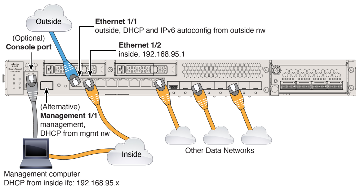
图 3. Secure Firewall 3100 的布线
