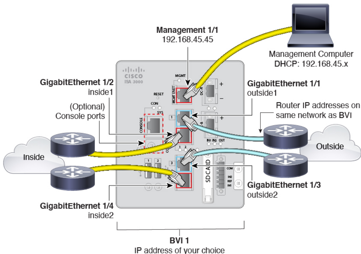
图 4: ISA 3000
