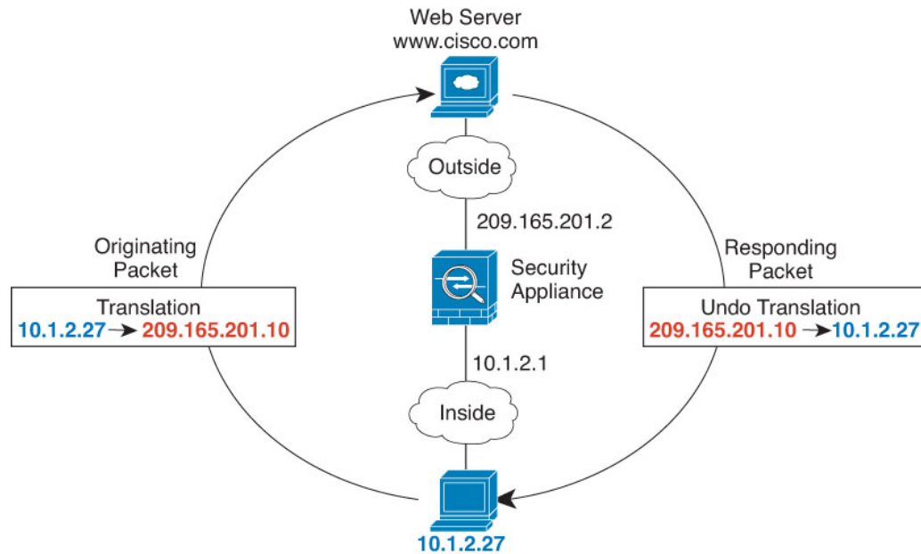
图 34: NAT 示例：路由模式
