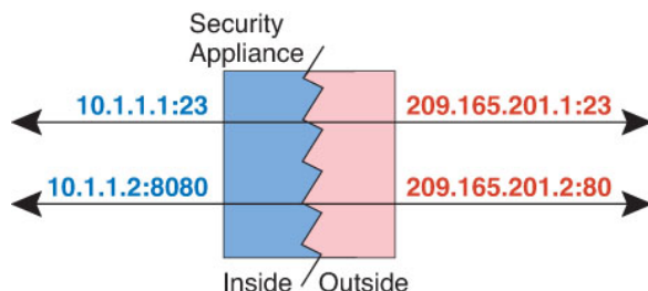
图 40: 支持端口转换的典型静态 NAT 场景
