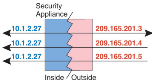
图 41: 一对多静态 NAT
