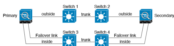
图 10: 使用安全交换机连接
