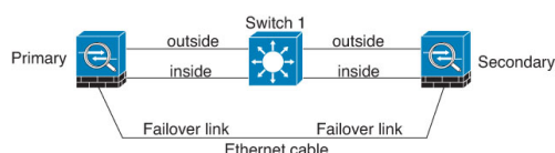
图 9: 通过电缆连接
