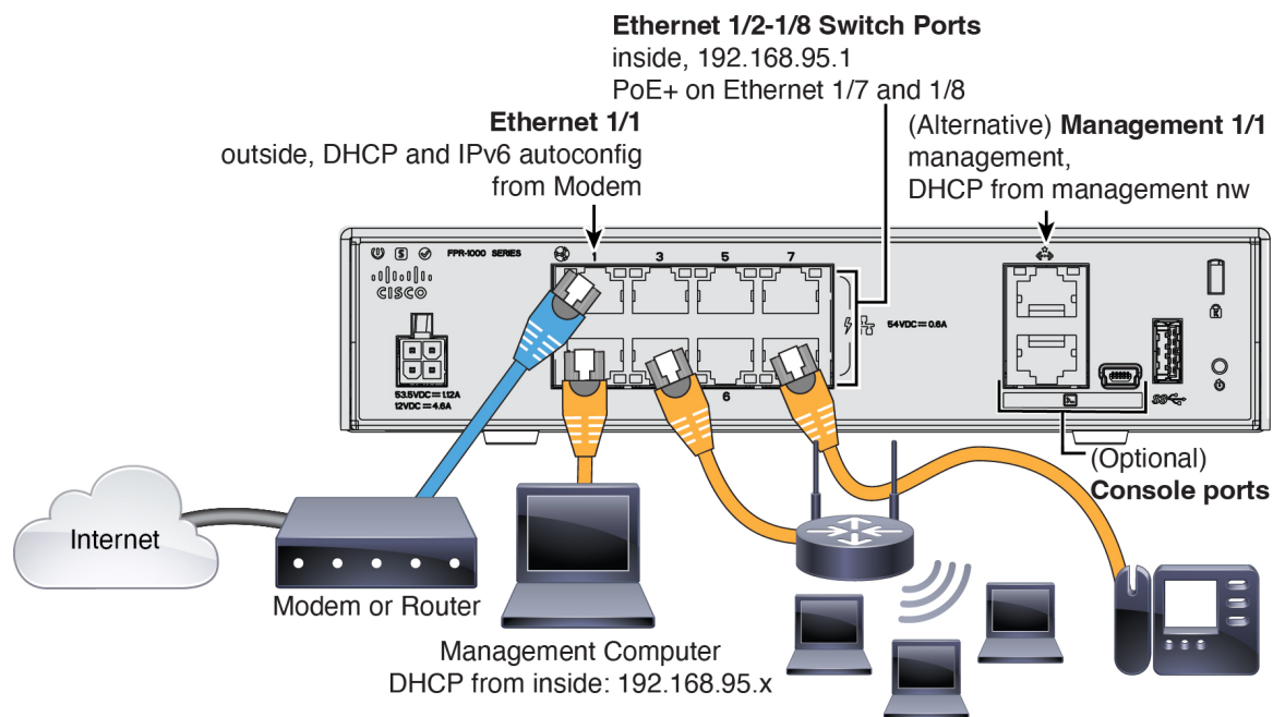
图 1: Firepower 1010 的布线
