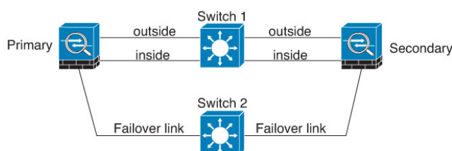
图 9: 通过电缆连接
