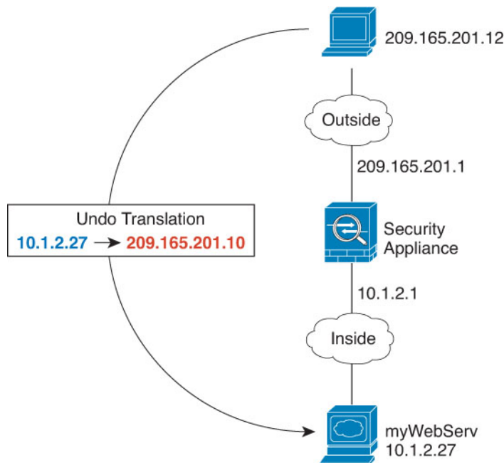
图 46: 面向内部 Web 服务器的静态 NAT
