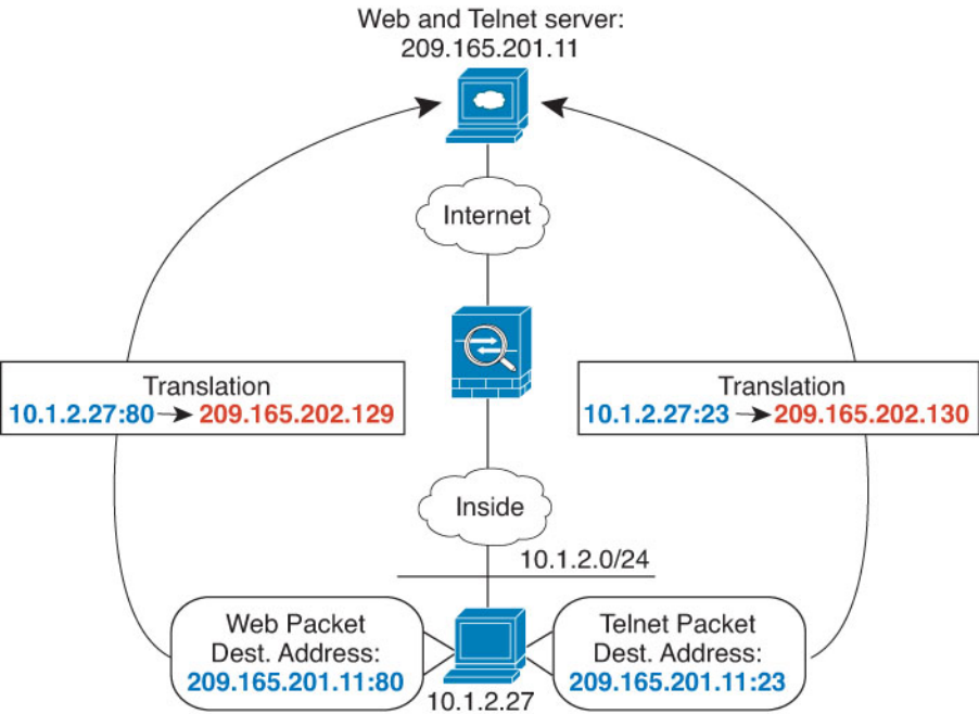
图 49: 具有不同目标端口的手动 NAT
