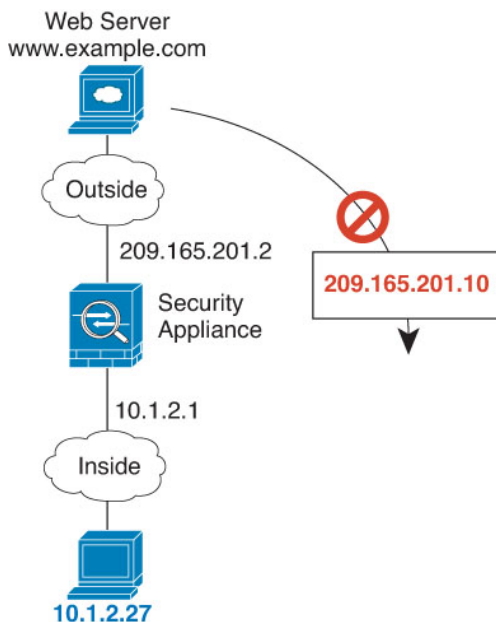
图 37: 远程主机尝试向映射地址发起连接
