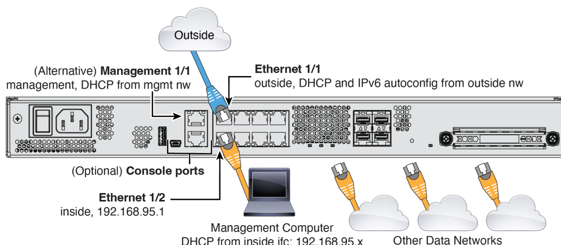
图 2: Firepower 1100 的布线
