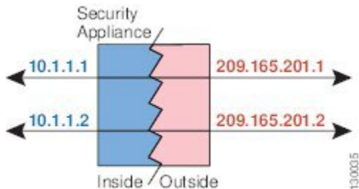
图 6: 静态 NAT
