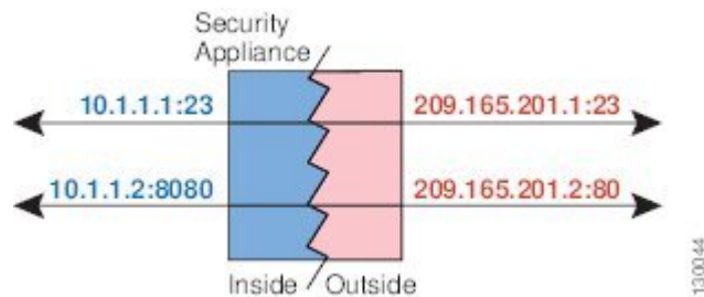
图 7: 支持端口转换的典型静态 NAT 场景
