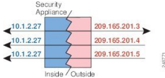
图 8: 一对多静态 NAT
