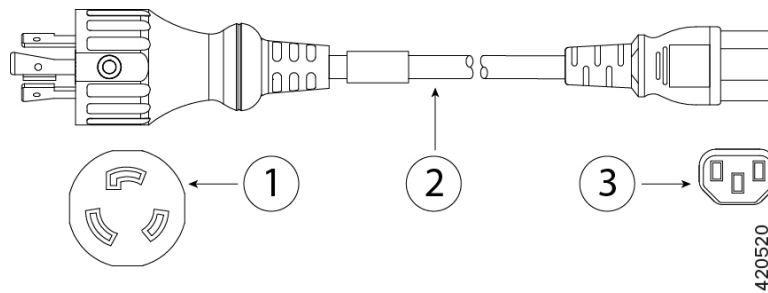
图 27: 日本 CAB-L620P-C13-JPN
