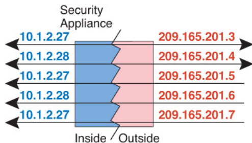
图 10: 少对多静态 NAT
