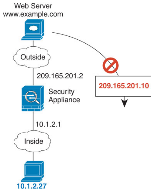
图 4: 远程主机尝试向映射地址发起连接
