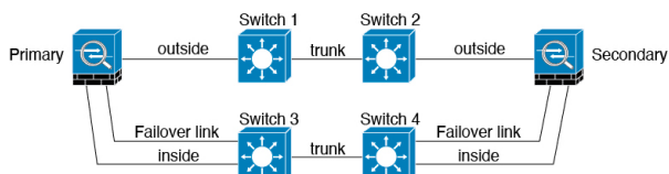
图 6: 使用安全交换机连接
