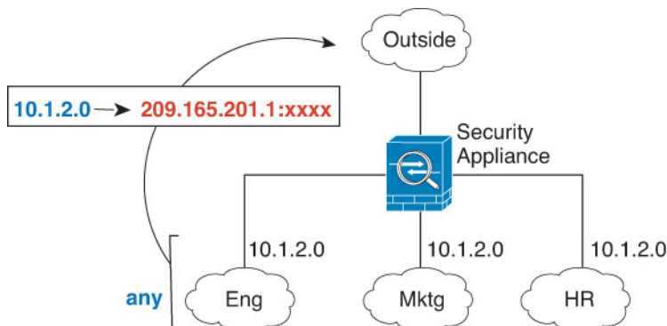
图 31: 指定任何接口
