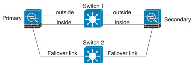
图 5: 通过电缆连接
