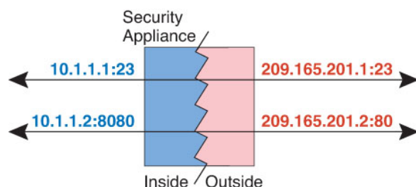
图 36: 支持端口转换的典型静态 NAT 场景
