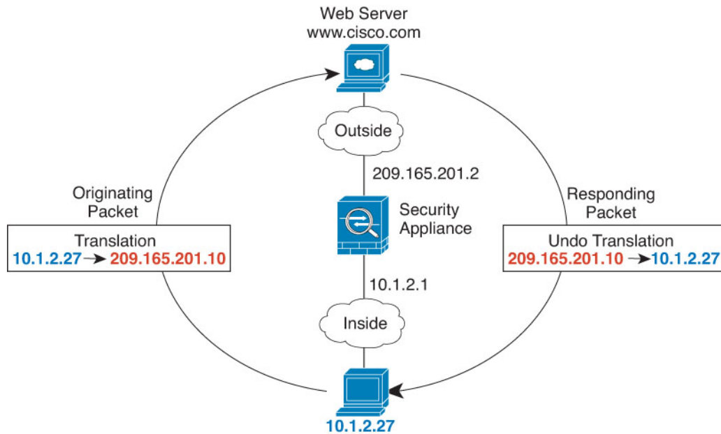
图 30: NAT 示例：路由模式
