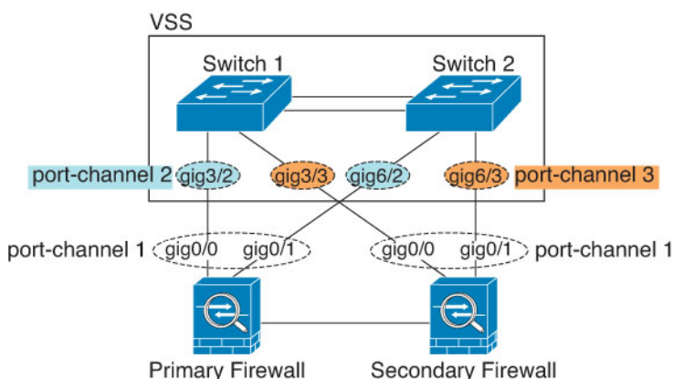
图 8: 主用/备用故障转移和 VSS/vPC
