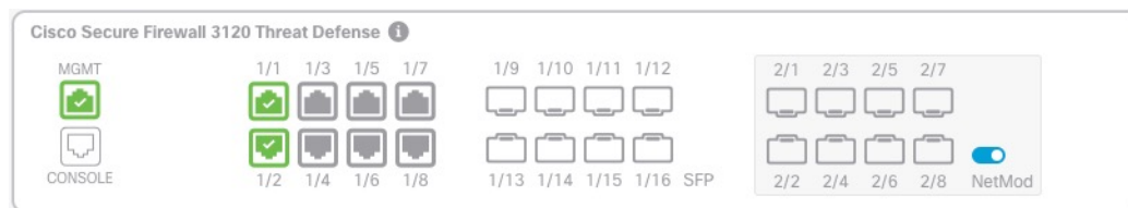
图 13: 禁用网络模块
