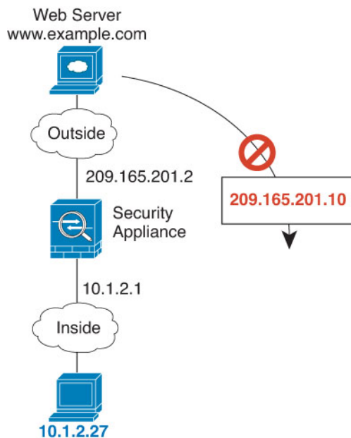
图 33: 远程主机尝试向映射地址发起连接
