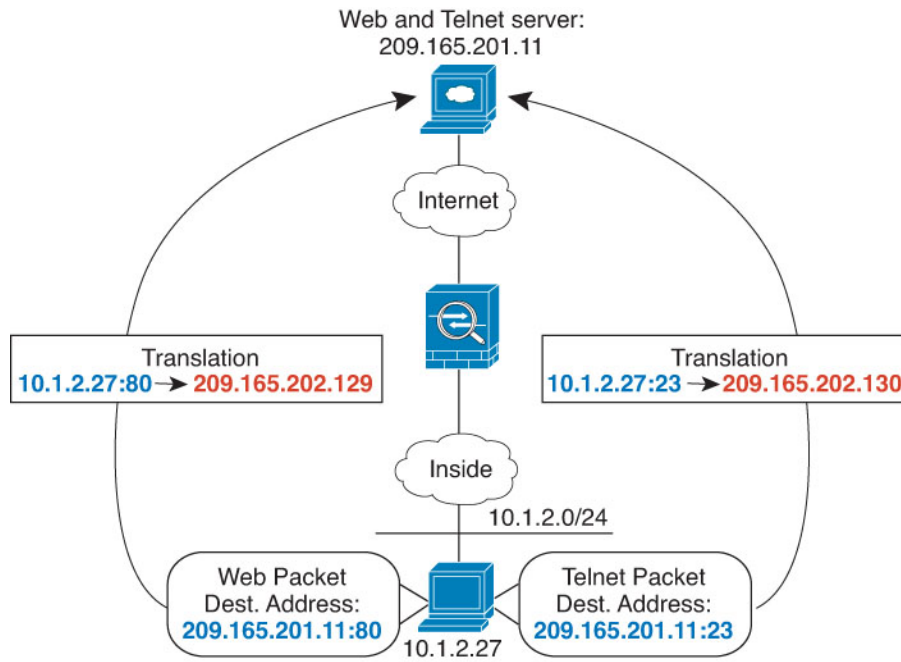
图 45: 具有不同目标端口的手动 NAT
