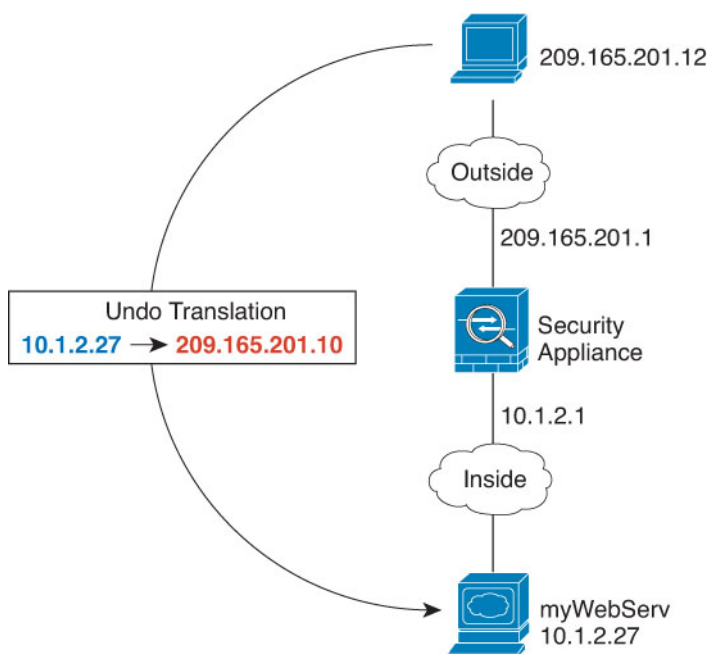
图 42: 面向内部 Web 服务器的静态 NAT
