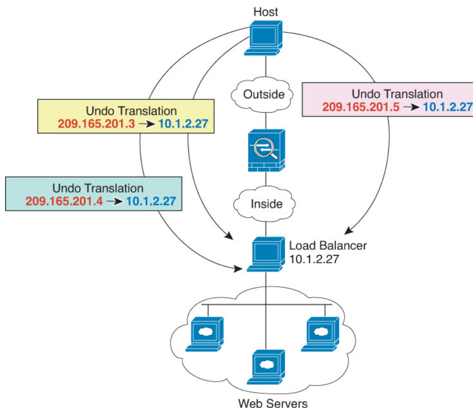
图 38: 一对多静态 NAT 示例
