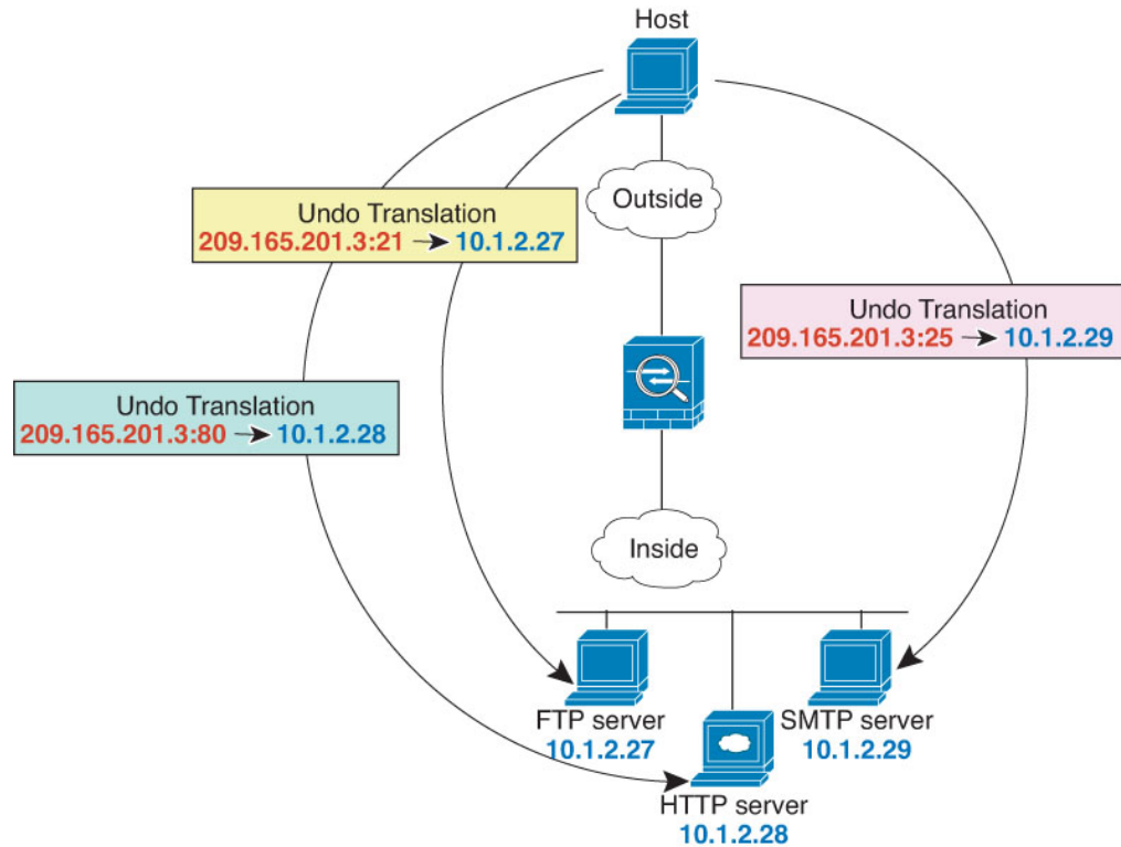
图 43: 支持端口转换的静态 NAT
