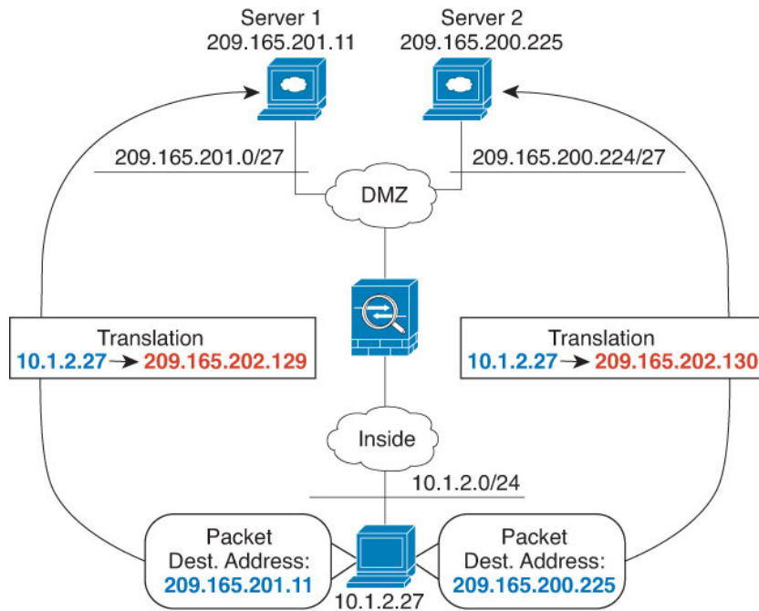
图 44: 具有不同目标地址的手动 NAT
