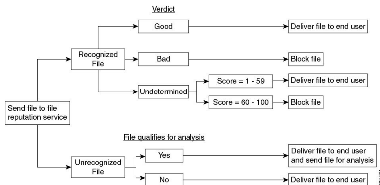
Figure 1: 面向公共云文件分析部署的思科高级恶意软件保护 工作流程
