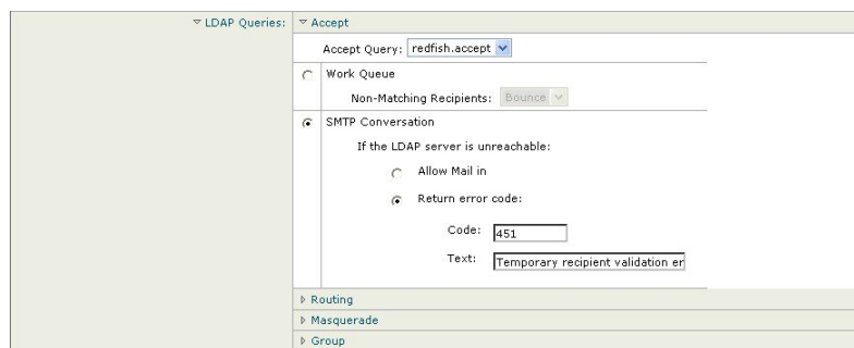
Figure 7: 配置 SMTP 会话期间的接受查询
