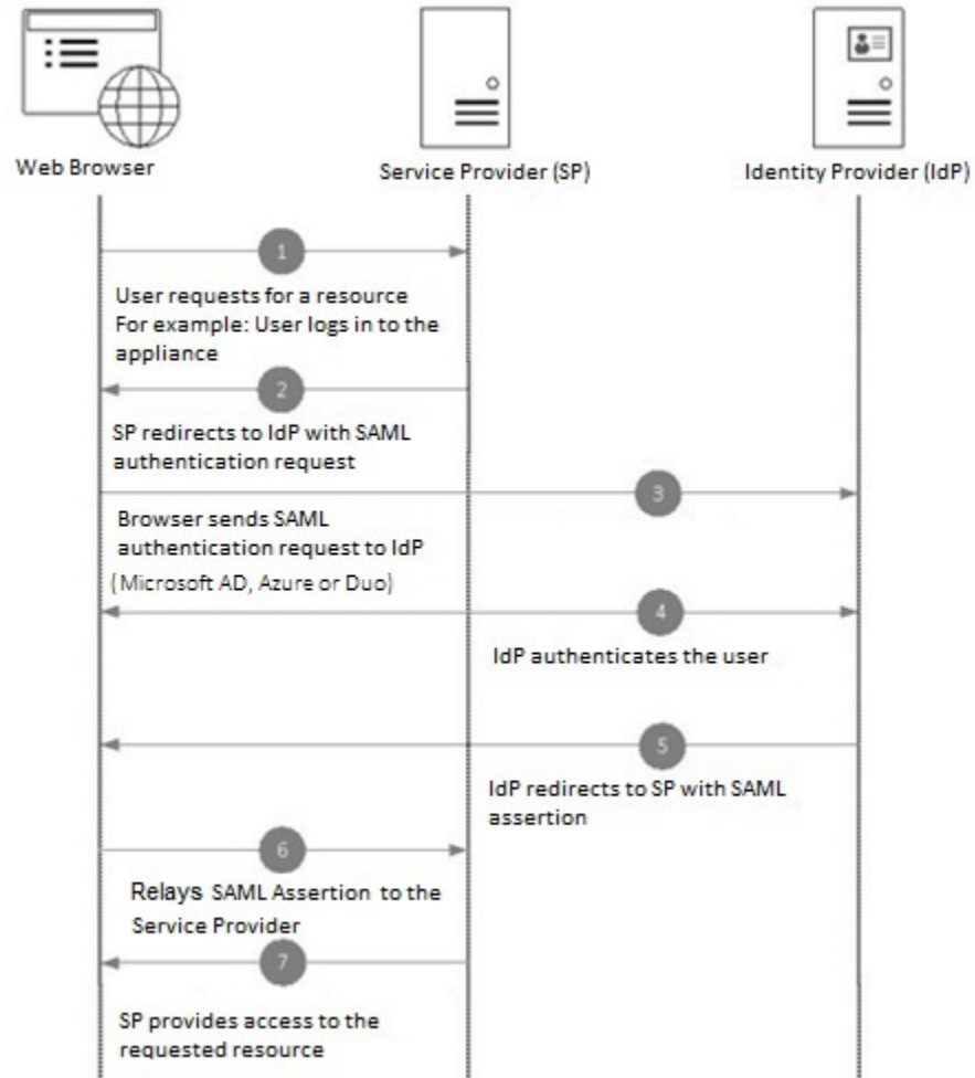
图 3: SAML workflow
