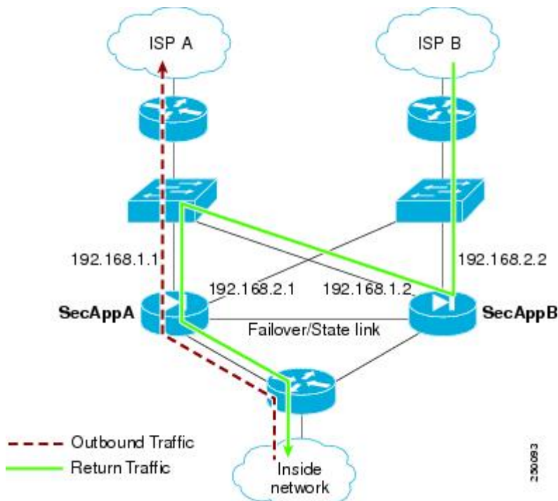
图 6: ASR 示例
