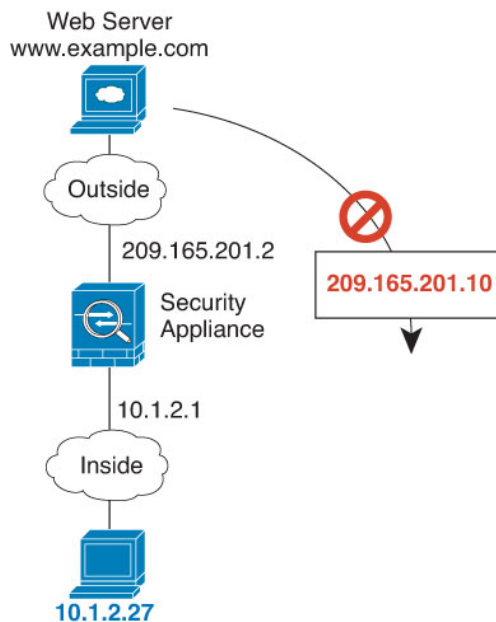
图 3: 远程主机尝试向映射地址发起连接
