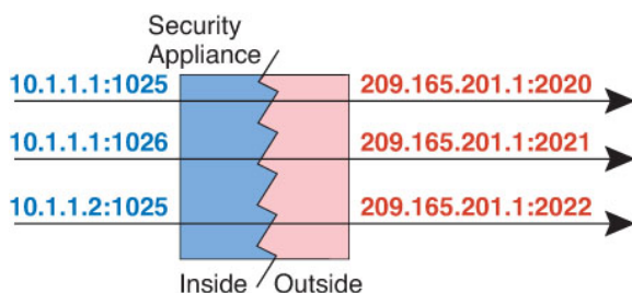
图 4: 动态 PAT
