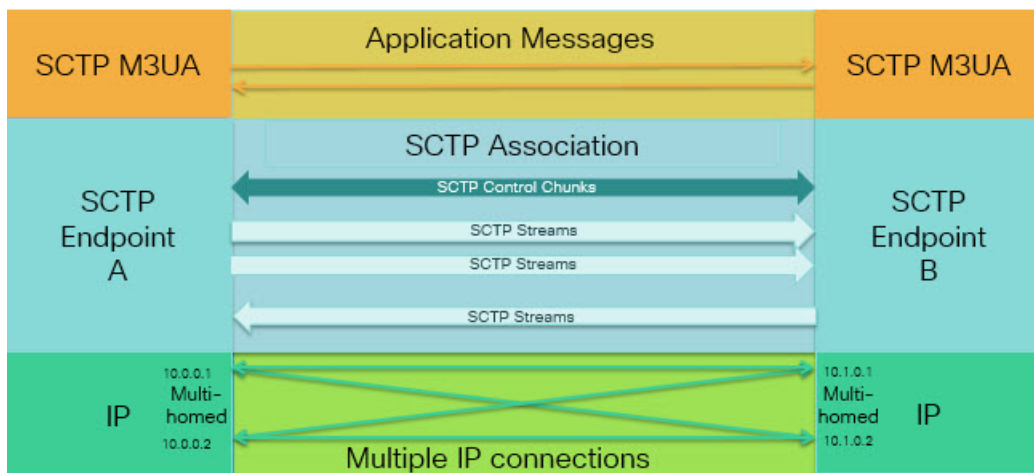
图 1: SCTP 关联与流之间的关系
