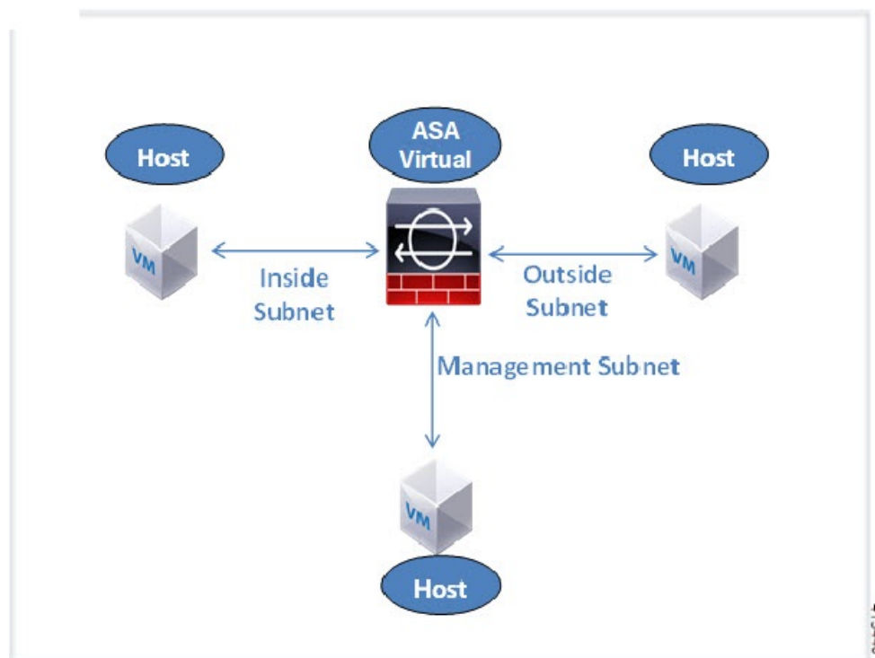
图 1: 在路由防火墙模式下建议用于 ASA Virtual 的网络拓扑
