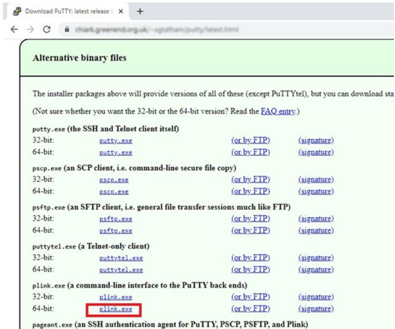
图 2: 下载 PuTTY
