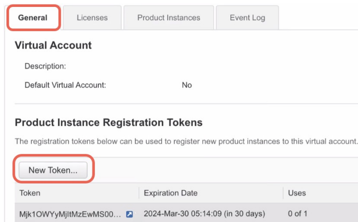
图 7: 新建令牌
