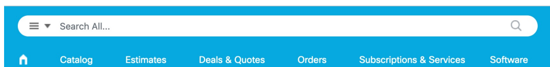
图 13: 许可证搜索
