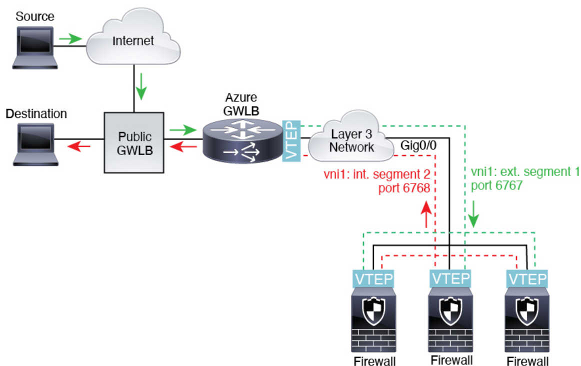
图 4: Azure 网关负载均衡器和配对代理
