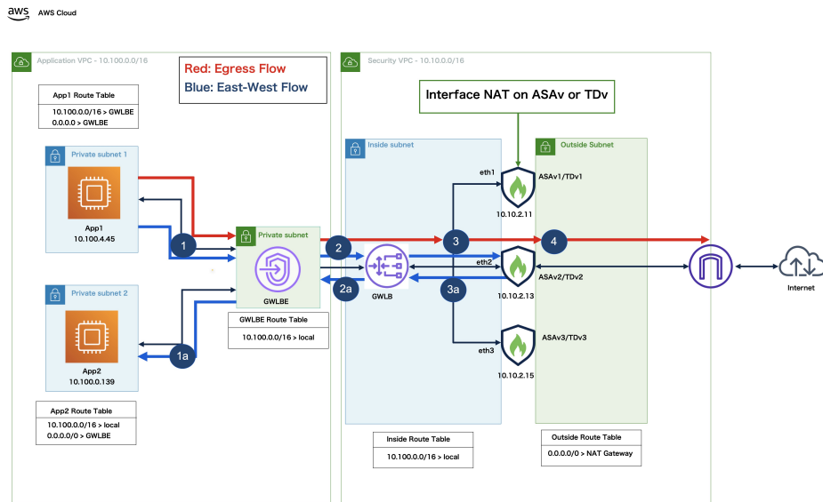
图 2: Geneve 双臂代理 - 来自单 VPC 的出口流量
