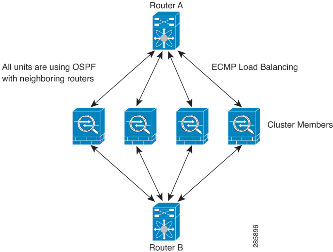
图 8: 独立接口模式下的动态路由
