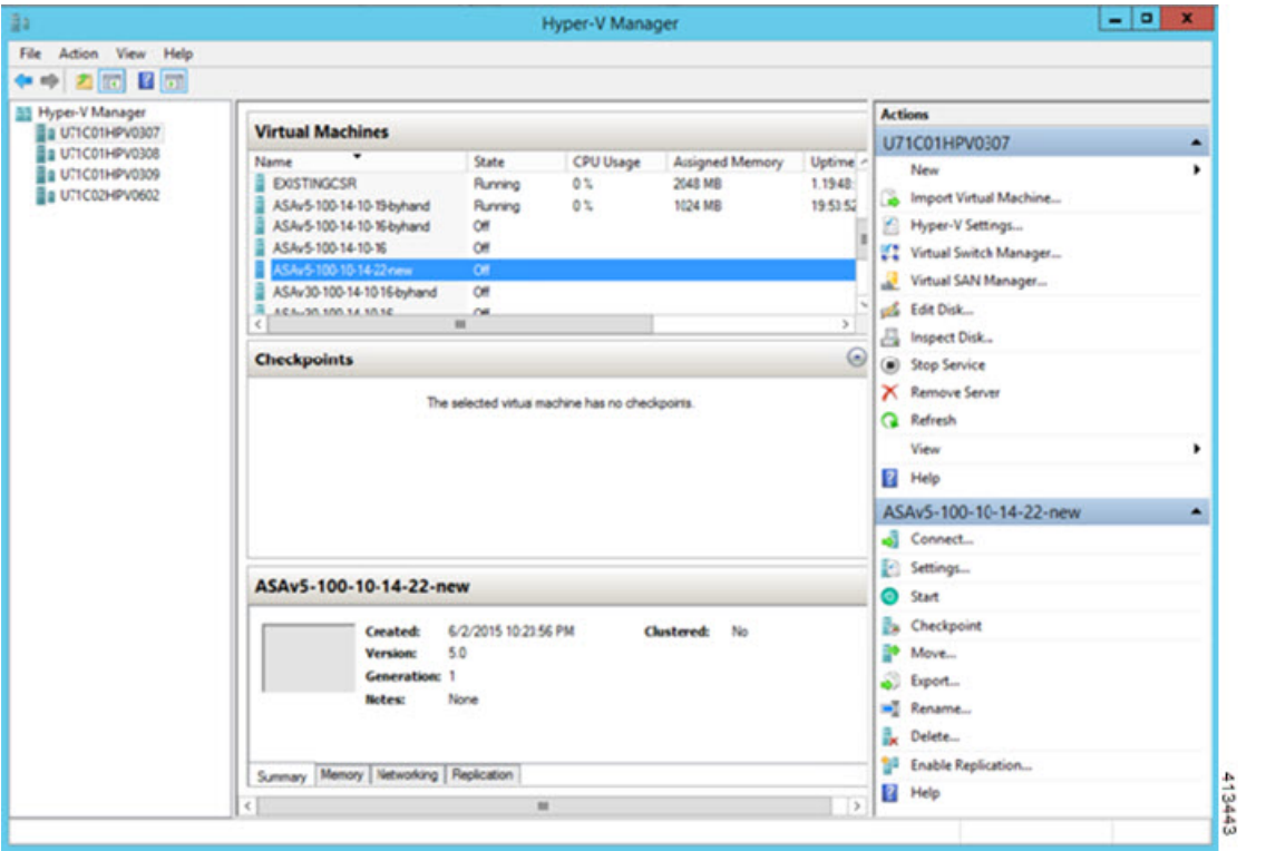
图 4: Hyper-V 管理器
