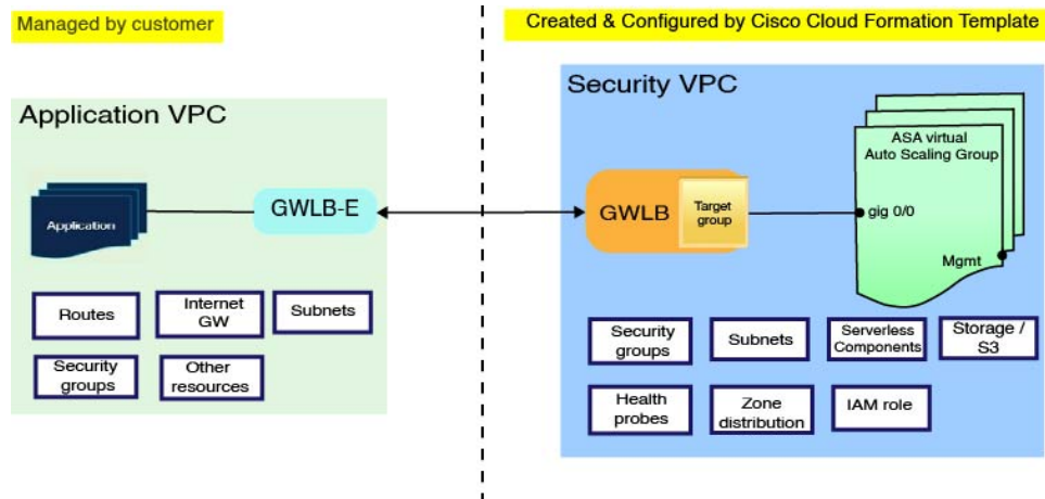
图 2: ASA Virtual AWS GWLB Auto Scale 使用案例图
