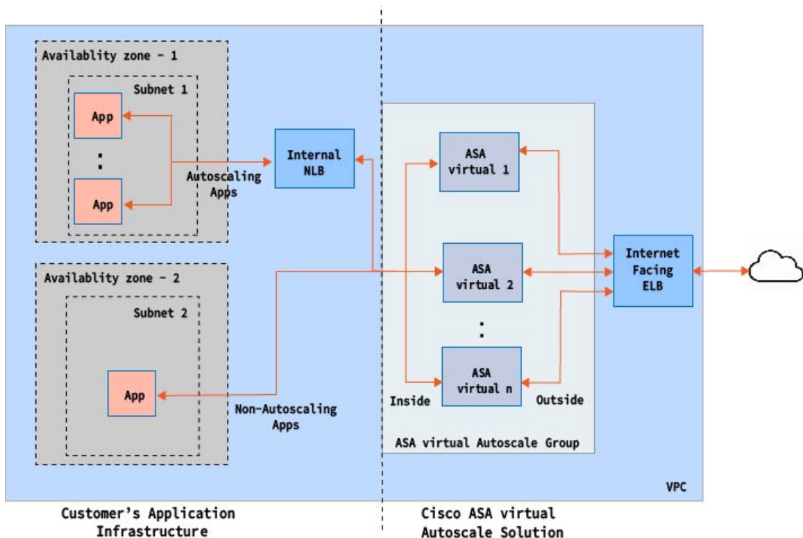
图 1: 使用三明治拓扑的 ASA Virtual Auto Scale 使用案例图
