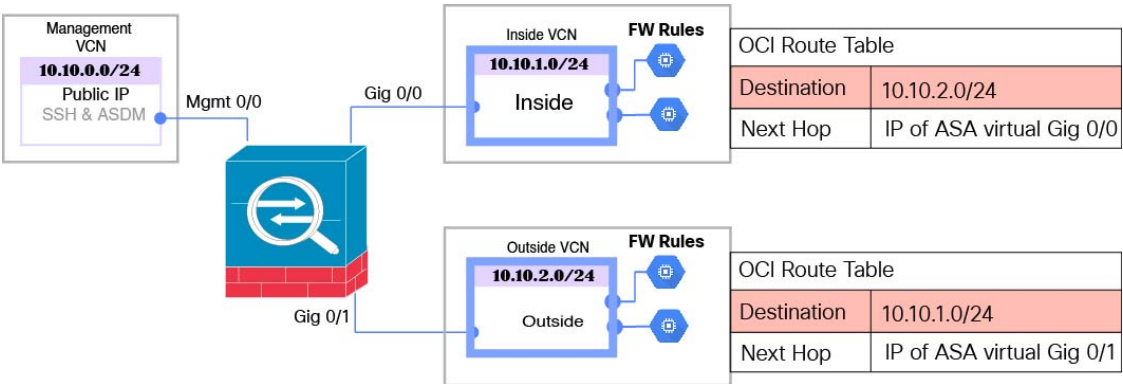
图 51: OCI 上的 ASA Virtual部署示例
