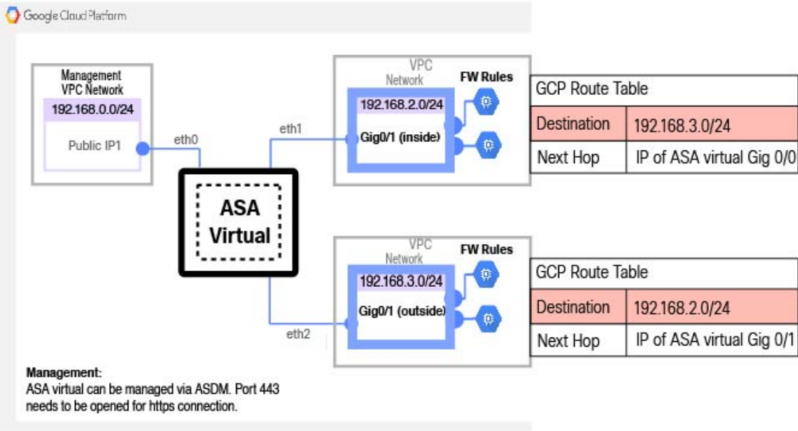
图 55: GCP 上的 ASA Virtual部署示例
