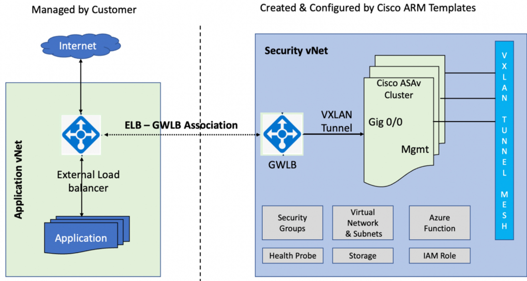
图 4: 具有 GWLB 的 Azure 上的 ASA 集群
