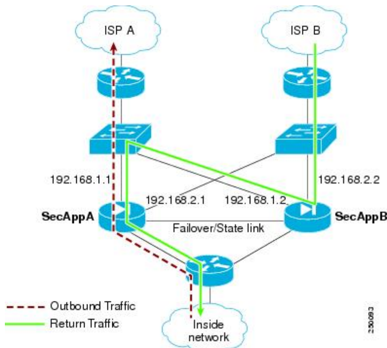
图 6: ASR 示例
