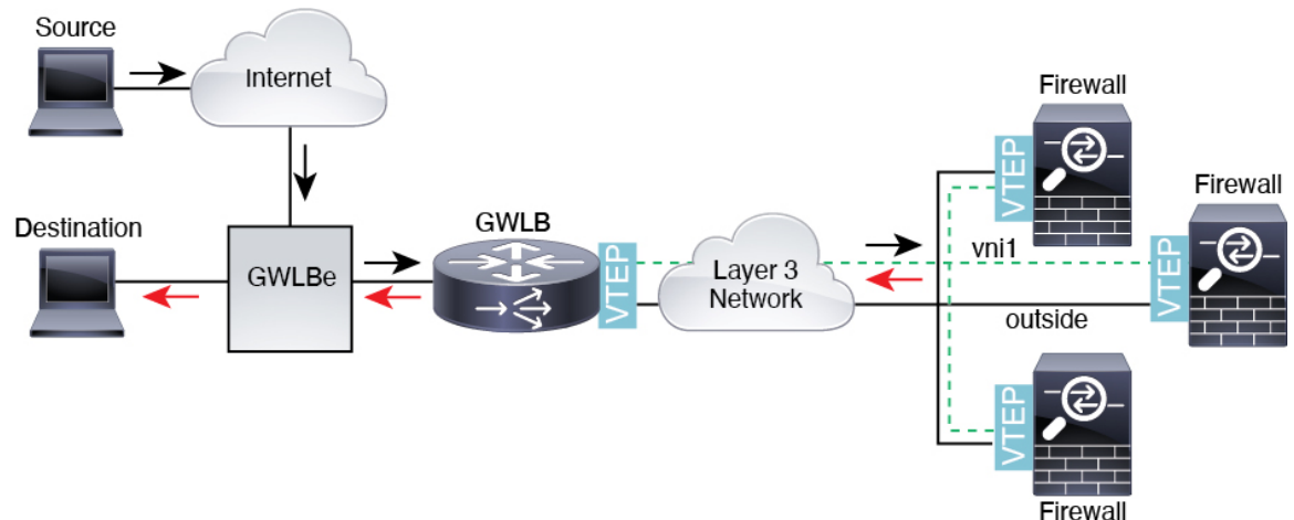
图 1: Geneve 单臂代理
