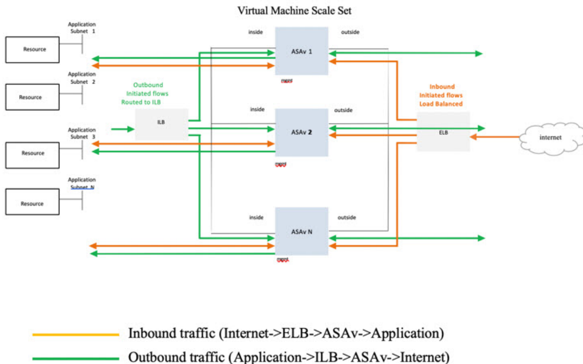
图 1: ASA Auto Scale 使用案例
