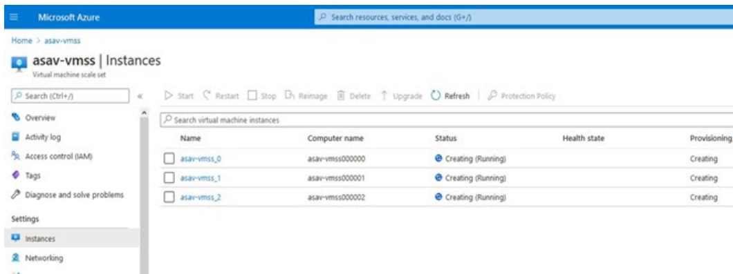
图 16: 正在运行的 ASAv 实例
