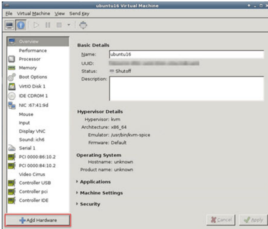
图 11: 添加硬件
