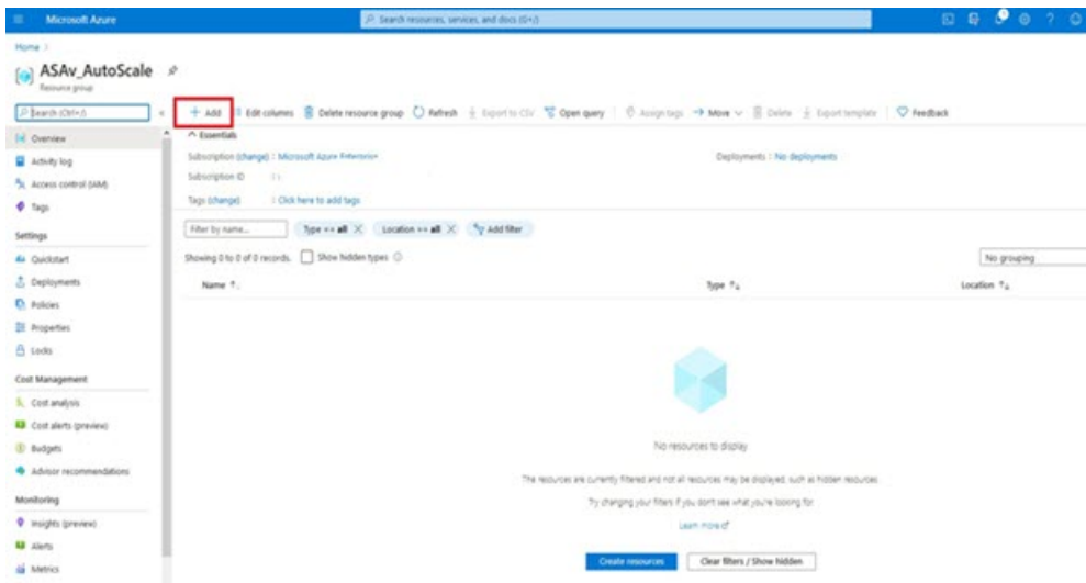
图 17: Azure 门户
