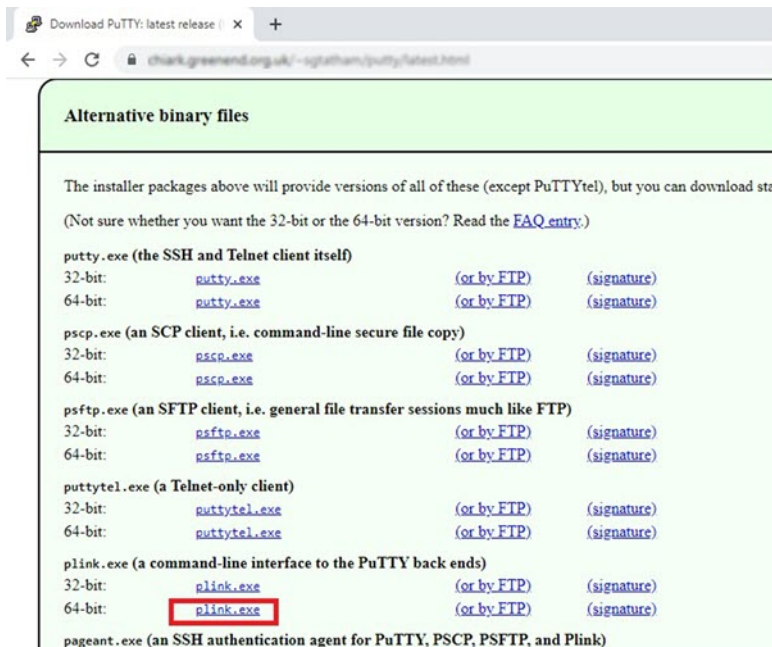
图 25: 下载 PuTTY
