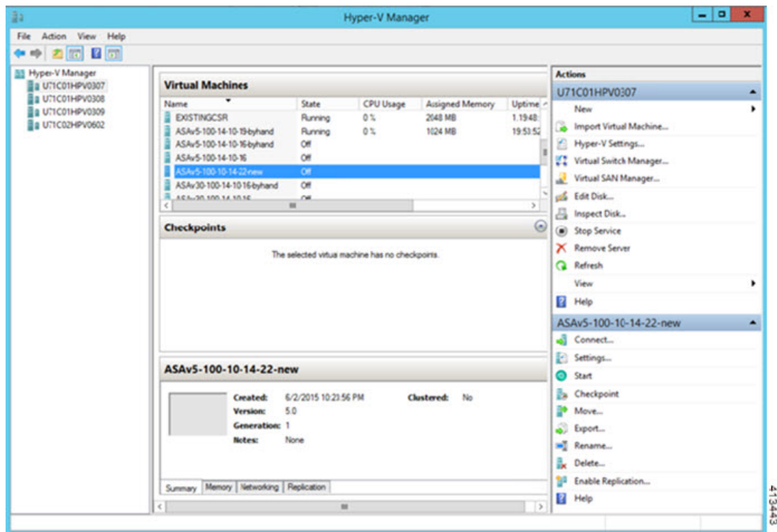
图 40: Hyper-V 管理器
