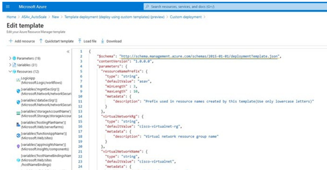
图 20: 编辑模板
