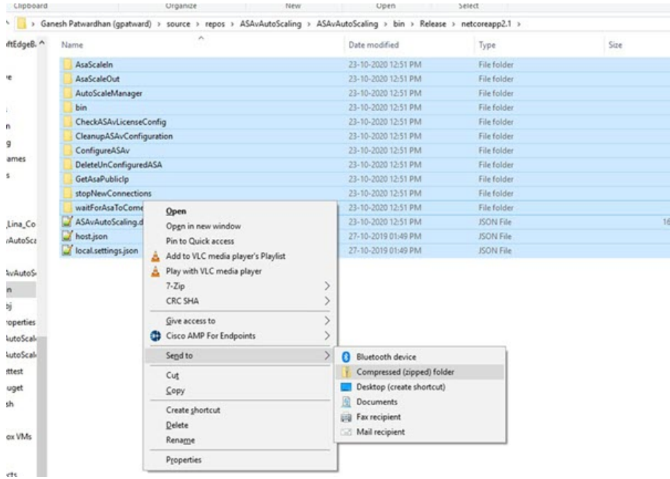
图 36: 生成 ASM_Function.zip
