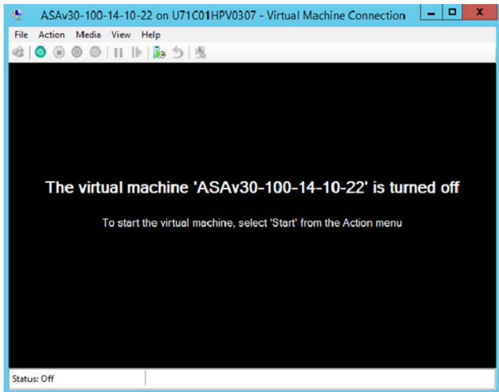
图 46: 启动虚拟机
