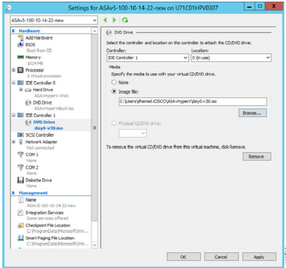
图 38: Hyper-V 管理器
