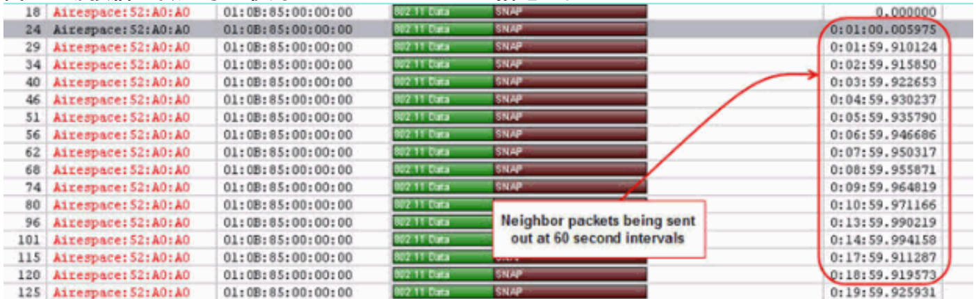
图 2：邻接信息传送每60秒对01:0B:85:00:00:00组播地址。
