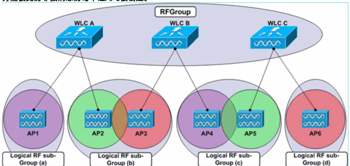
图 6：在本例中，连接到 WLC A 和 C 的 AP 无法侦听到彼此的邻居消息。WLC B 可以同时侦听到 WLC A 和 C，并因此可以与二者共享另一方的信息，以便随后形成一个 RF 组。分离逻辑 RF 小群为能彼此的邻接消息的每个组 APs 被创建。
