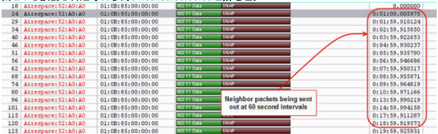
图 2：邻接信息传送每60秒对01:0B:85:00:00:00组播地址。
