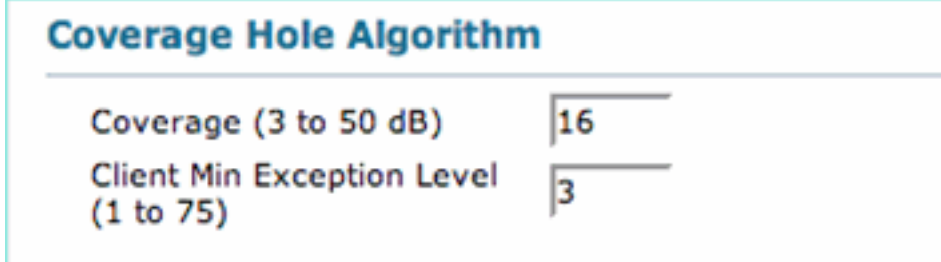
图 19：覆盖空洞部分，与配置文件阈值分离，提供大多数安装的默认值的最佳结果
