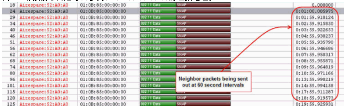
图 2：邻接信息传送每60秒到01:0B:85:00:00:00的组播地址。
